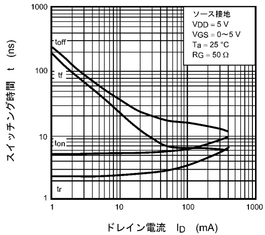
図 8.10 t - I_D
