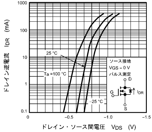
図 8.8 I_{DR} - V_{DS}
