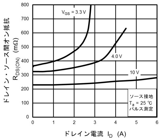
図 7.6 R_{DS(ON)} - I_D
