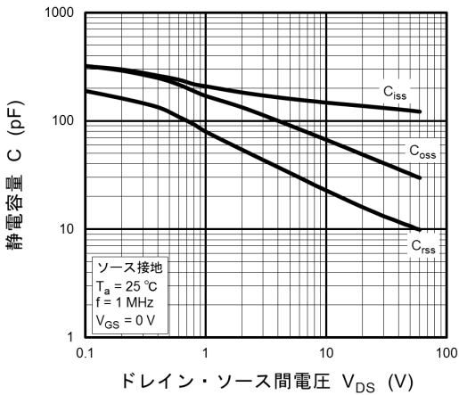
図 7.11 C - V_{DS}
