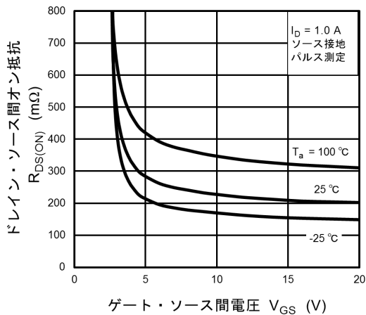
図 7.5 R_{DS(ON)} - V_{GS}
