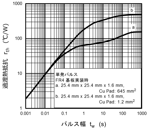
図 7.13 r_{th} - t_w
