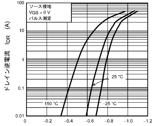
図 8.8 I_{DR} - V_{DS}
