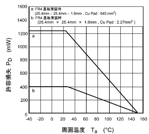
図 8.12 P_D - T_a
