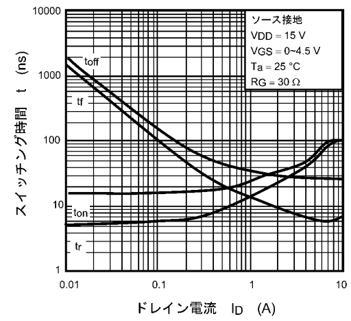
図 8.10 t - I_D
