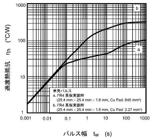
図 8.12 r_{th} - t_w
