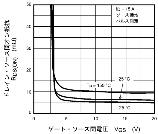
図 8.4 R_{DS(ON)} - V_{GS}
