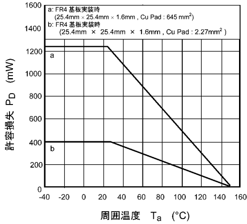
図 8.13 P_D - T_a
