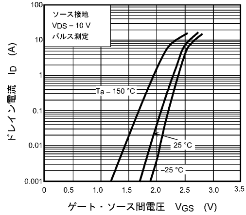
図 8.2 I_D - V_{GS}
