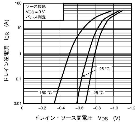
図 8.8 I_{DR} - V_{DS}
