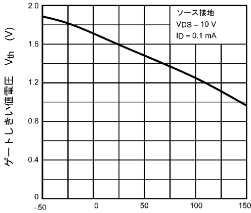
図 8.7 V_{th} - T_a
