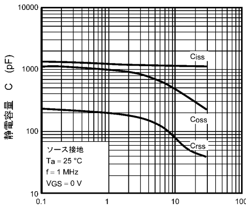
図 8.9 C - V_{DS}
