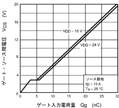
図 8.11 ダイナミック入力特性
