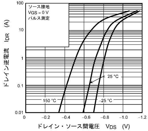
図 8.8 I_{DR} - V_{DS}
