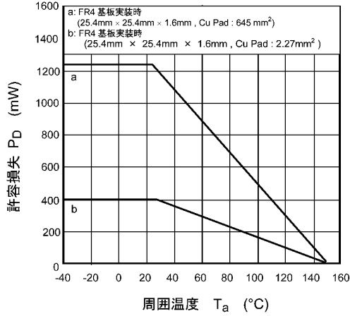
図 8.13 P_D - T_a
