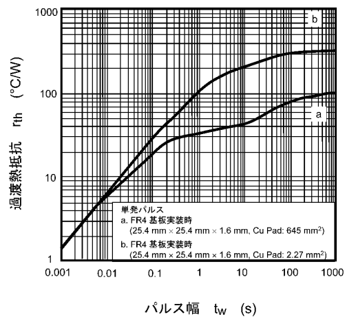
図 8.12 r_{th} - t_w
