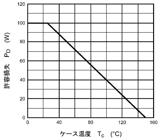
ケース温度 T_c (°C) 図 8.15 P_D - T_c (最大値 (保証値))
