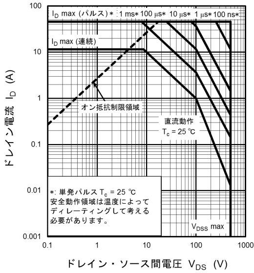
図 8.17 安全動作領域 (最大値 (保証値))
