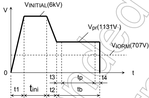
ダイアグラム 1 EN 60747 による試験電圧波形、手順 a)、破壊試験 (型式試験や抜き取り試験に適用) Figure 1 Partial discharge measurement procedure according to EN 60747 Destructive test for qualification and sampling tests.
