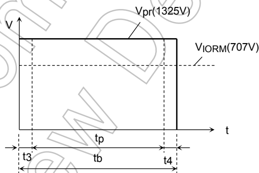
ダイアグラム 2 EN 60747 による試験電圧波形、手順 b)、非破壊試験 (全数試験に適用) Figure 2 Partial discharge measurement procedure according to EN 60747 Non-destructive test for 100% inspection.
