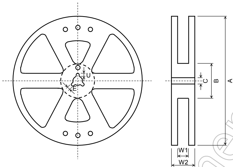
図 4 リール形状
