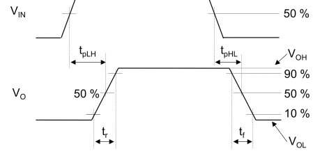
図 12.1.5 伝搬遅延時間測定回路, 波形
