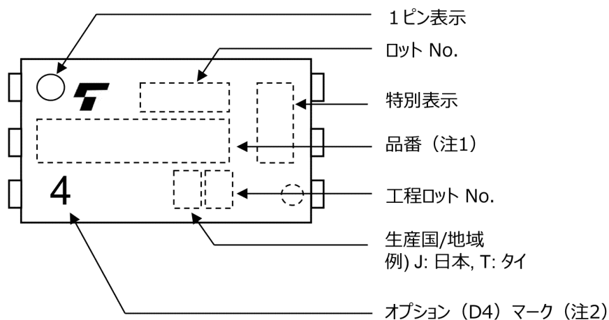
図 16.4 現品表示例
