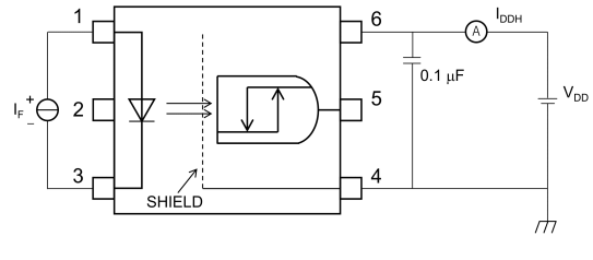
図 12.1.4 IDD_H測定回路
