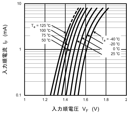
図 12.2.1 I_F - V_F
