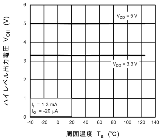
図 12.2.5 V_{OH} - T_a
