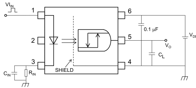
図 12.1.5 伝搬遅延時間測定回路, 波形
