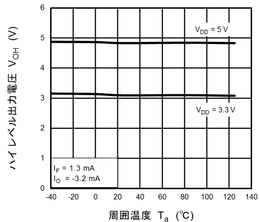
図 12.2.6 V_{OH} - T_a
