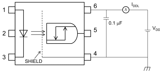
図 12.1.3 IDD_L測定回路
