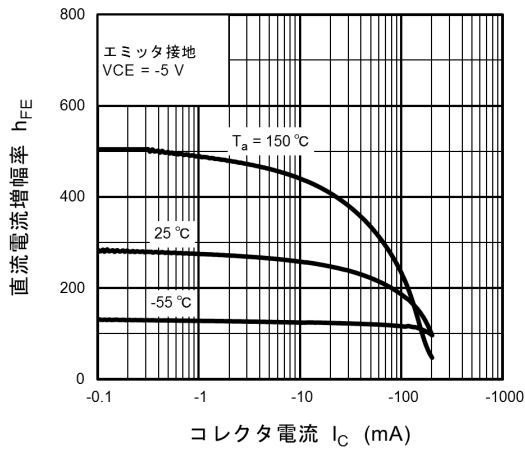
図 6.1 h_{FE} - I_C
