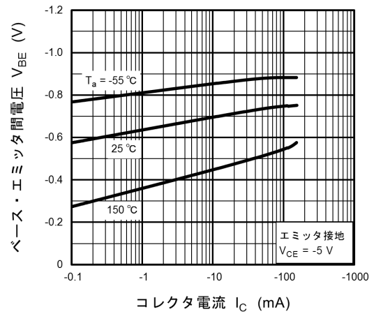
図 6.2 V_{BE} - I_C
