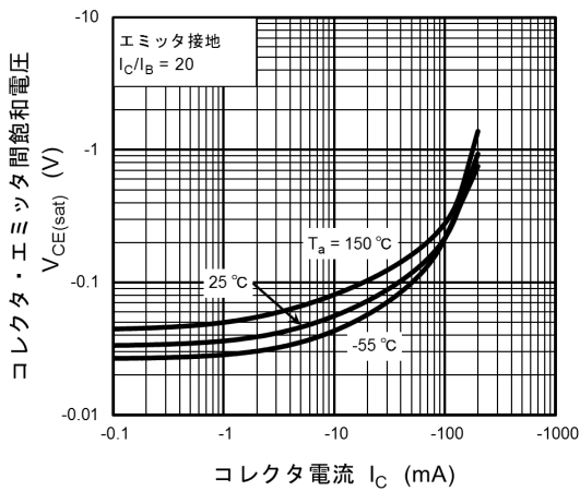
図 6.3 V_{CE(sat)} - I_C
