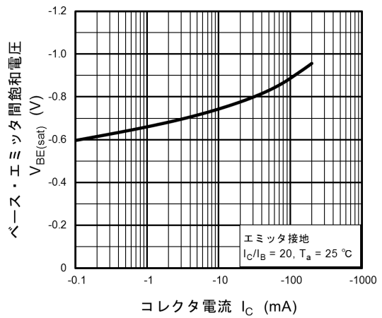
図 6.4 V_{BE(sat)} - I_C
