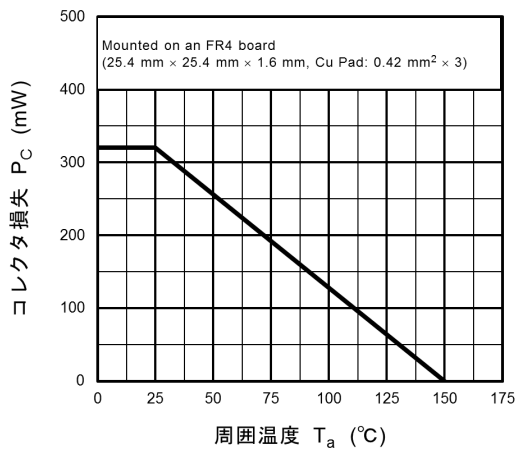
図 6.5 P_C - T_a
