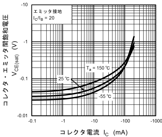
図 6.3 V_{CE(sat)} - I_C
