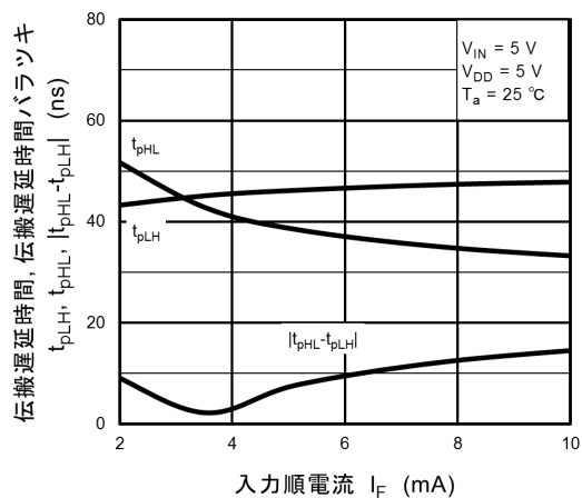
図 12.2.13 t_{pLH} , t_{pHL} , |t_{pHL} - t_{pLH}| - I_F
