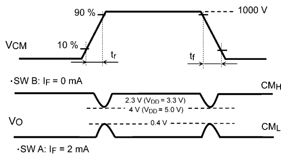
図 12.1.6 コモンモード過渡耐性測定回路, 波形
