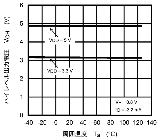
図 12.2.6 V_{OH} - T_a
