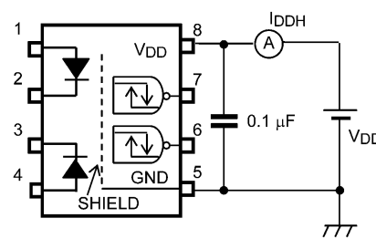
図 12.1.4 IDD H測定回路
