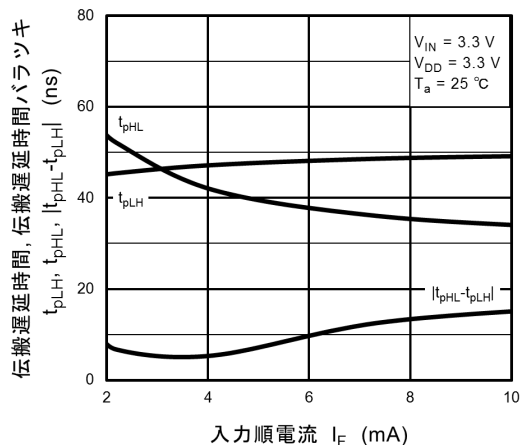
図 12.2.12 t_{pLH}, t_{pHL}, |t_{pHL} - t_{pLH}| - I_F
