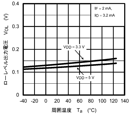
図 12.2.4 V_{OL} - T_a
