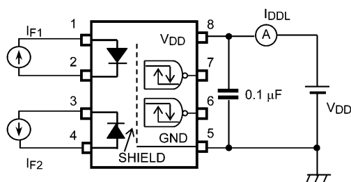
図 12.1.3 IDD L測定回路
