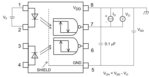
Fig. 12.1.2 V_{OH} Test Circuit
