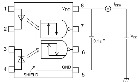
Fig. 12.1.4 I_{DDH} Test Circuit
