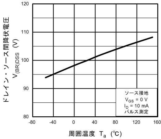
図 8.7 V_{(BR)DSS} - T_a
