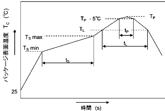
図 13.1.1 鉛フリーはんだ使用時の温度プロフィール例
