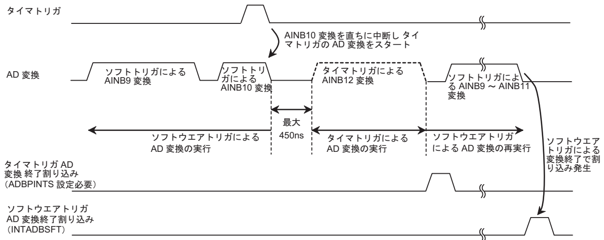
図 14-8 ソフトウェア AD 変換中のタイマ トリガ発生
