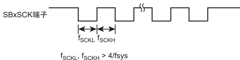
図 13-14 外部クロック入力時の最大転送周波数
