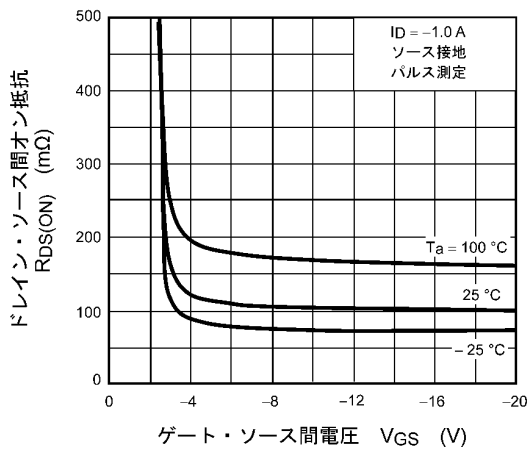
図 7.3 R_{DS(ON)} - V_{GS}
