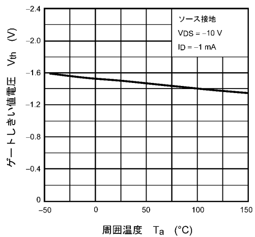
図 7.6 V_{th} - T_a
