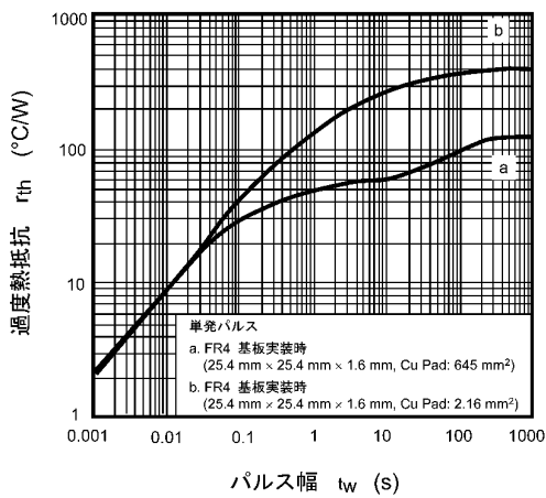
図 7.11 r_{th} - t_w
