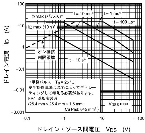
図 7.12 安全動作領域
