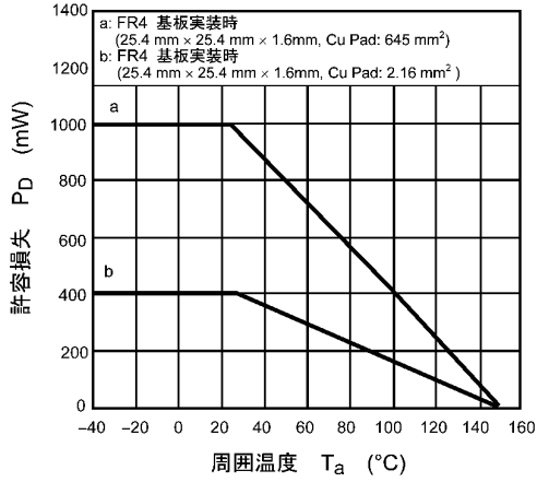
図 9.13 P_D - T_a
