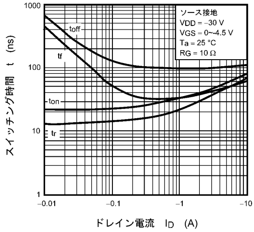
図 7.10 t - I_D
