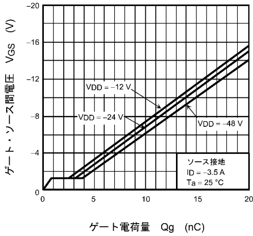
図 7.9 ダイナミック入力特性
