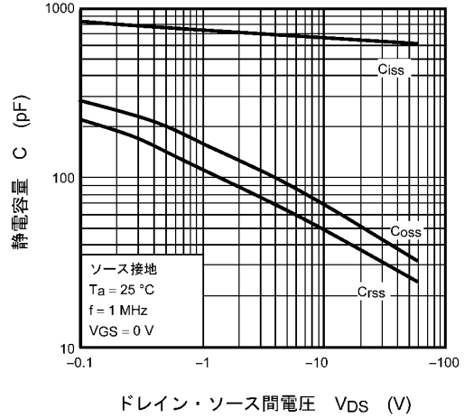
図 7.8 C - V_{DS}
