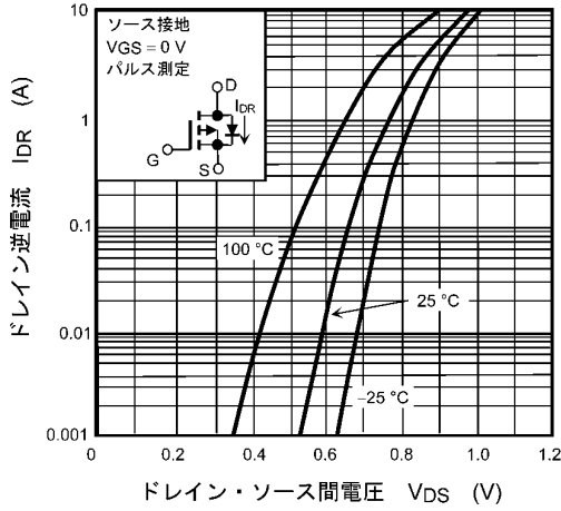
図 7.7 I_{DR} - V_{DS}
