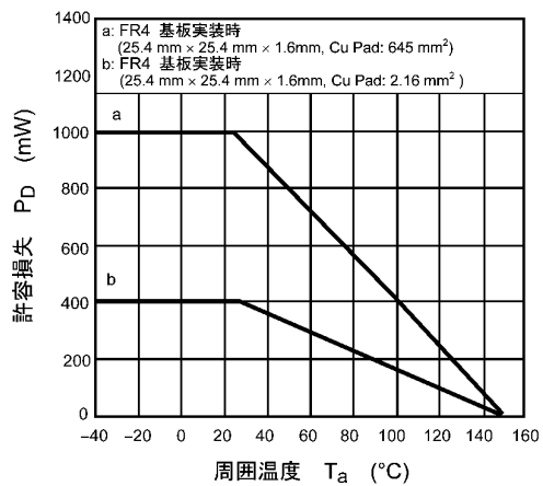
図 7.13 P_D - T_a
