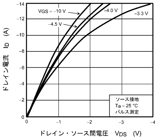
図 7.1 I_D - V_{DS}
