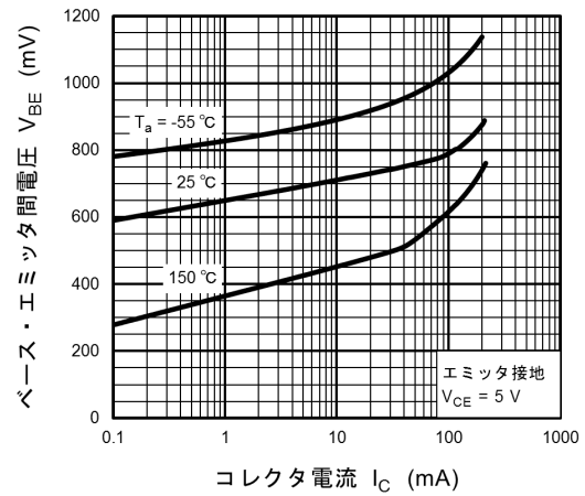
図 6.2 V_{BE} - I_C
