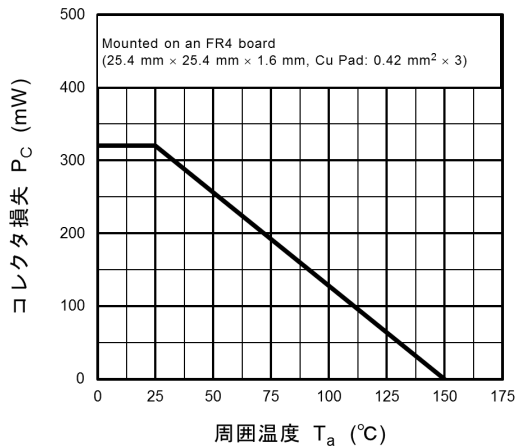
図 6.5 P_C - T_a
