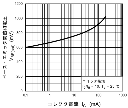
図 6.4 V_{BE(sat)} - I_C
