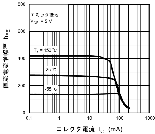
図 6.1 h_{FE} - I_C
