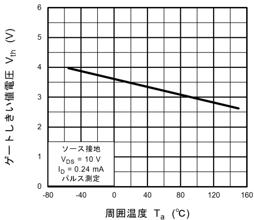
図 8.11 V_{th} - T_a
