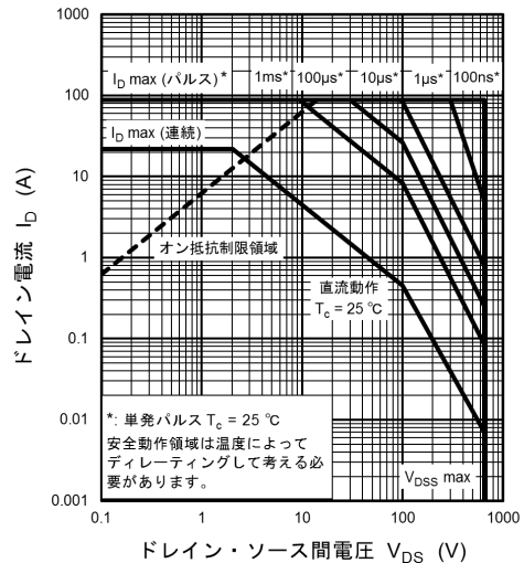
図 8.17 安全動作領域 (最大値 (保証値))
