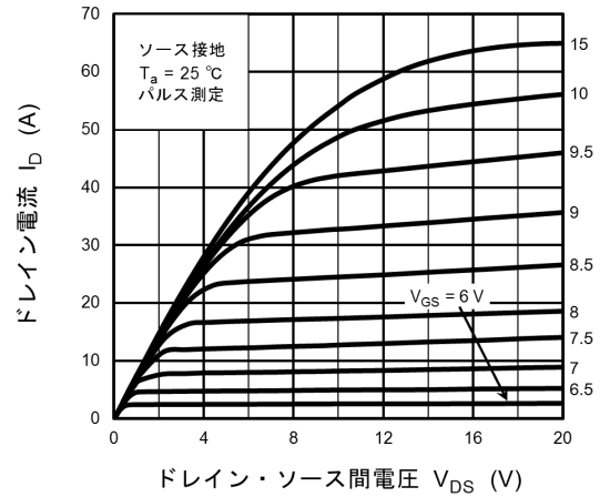
図 8.2 I_D - V_{DS}
