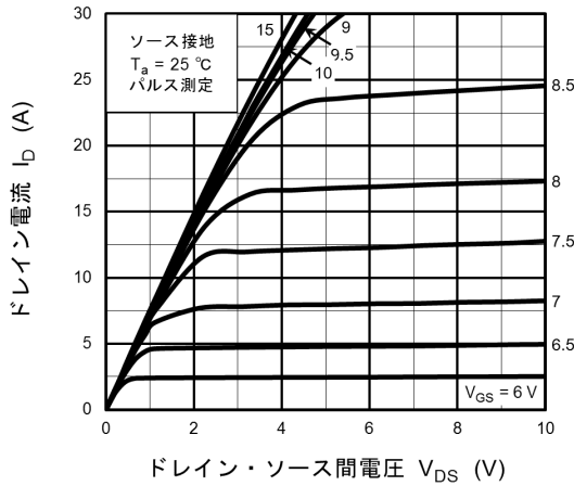
図 8.1 I_D - V_{DS}
