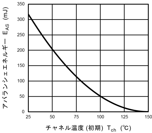
チャネル温度 (初期) T_{ch} (°C) 図 8.14 E_{AS} - T_{ch} (最大値 (保証値))
