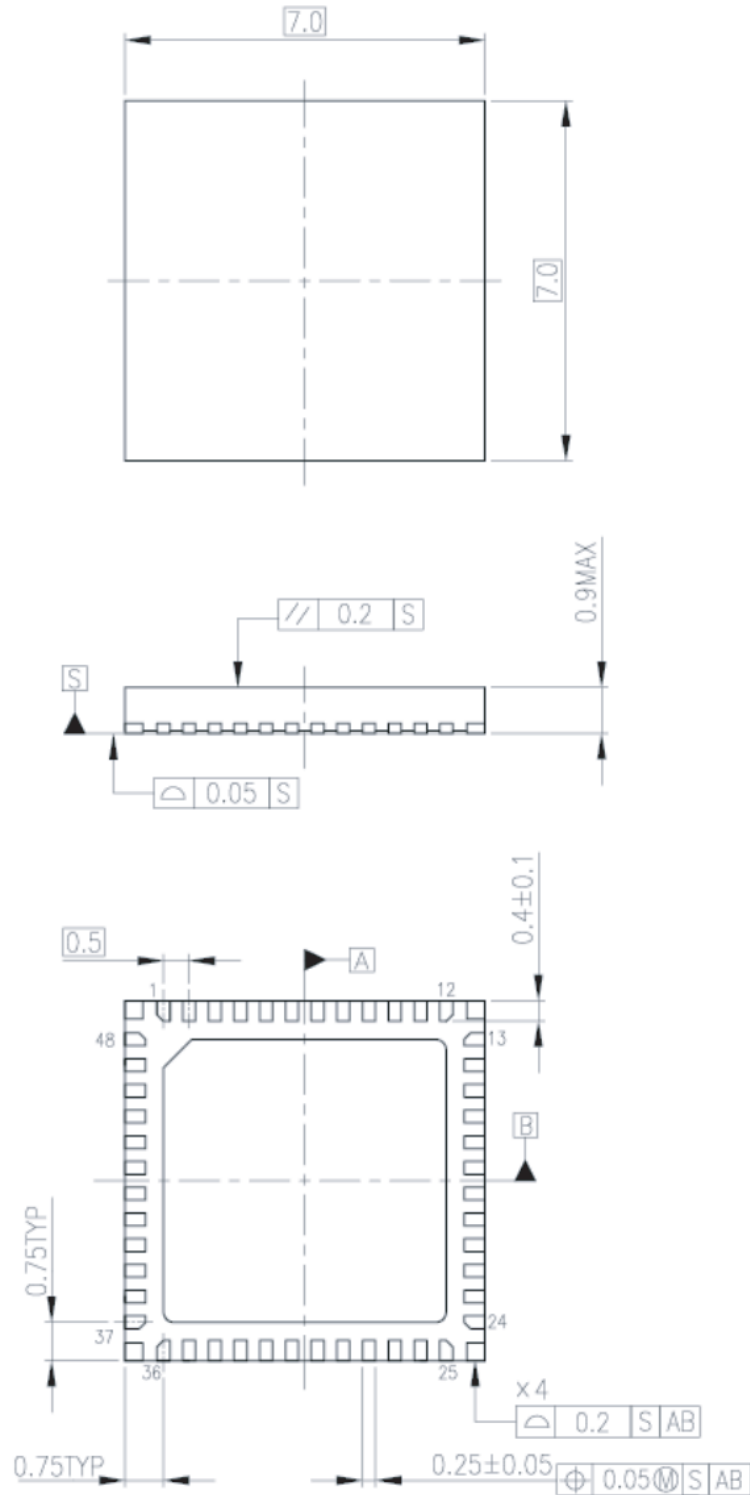
図 24-2 TMPM067FWQG
