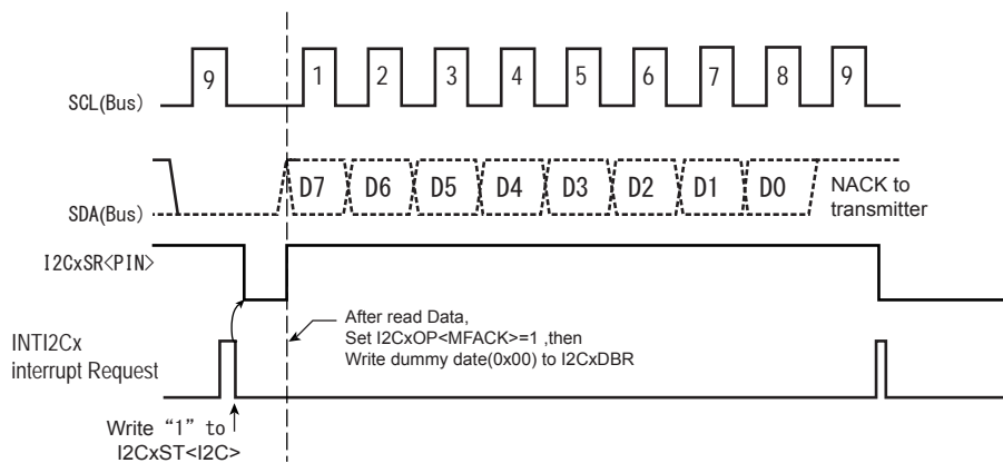
図 14-20 マスタレシーバモード時、データの送信を終了させるときの処理
