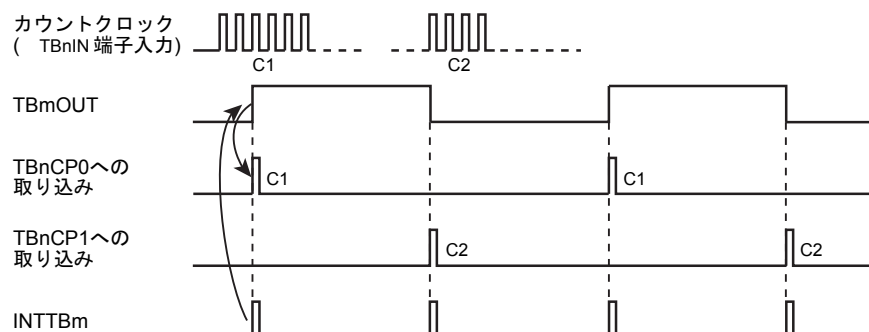
図 10-6 周波数測定
