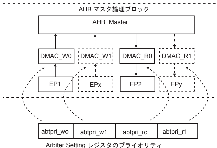
図 16-8 DMAC とプライオリティ領域の関係
