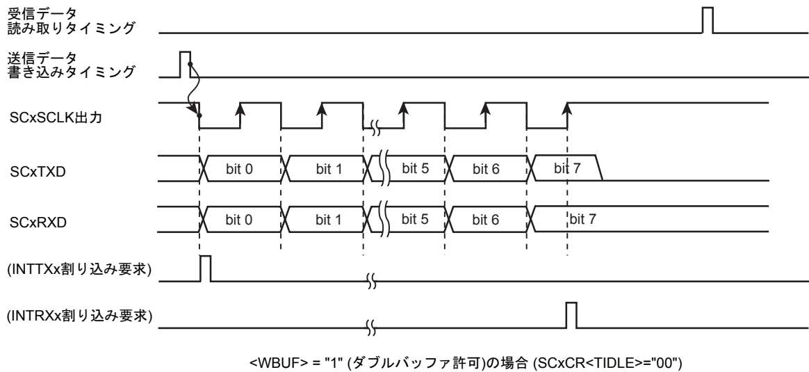
図 13-19 I/O インタフェースモード送受信動作(クロック出力モード)
