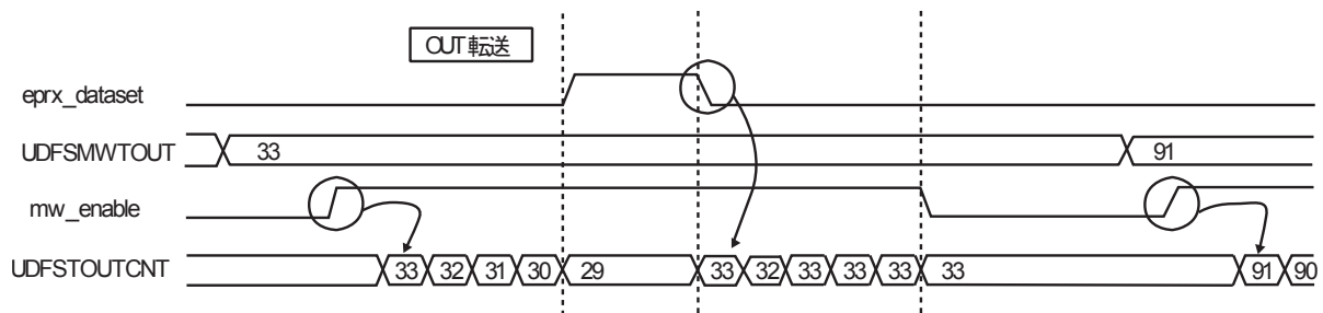
図 16-15 MW タイムアウトカウンタ例
