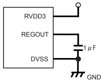
図 1-5 レギュレータ用コンデンサ接続図
