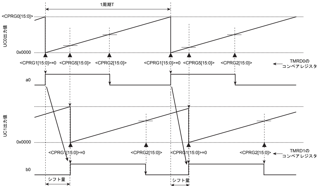
図 12-14 0 相(PPG0)と 1 相(PPG10)の位相関係例
