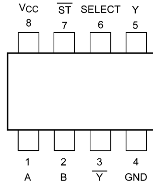
端子配置図 (Top view)
