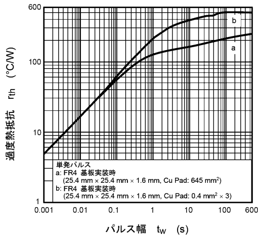
図 8.11 r_{th} - t_w
