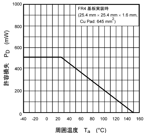
図 8.12 P_D - T_a
