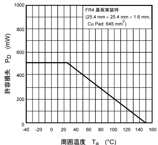
図 7.12 P_D - T_a
