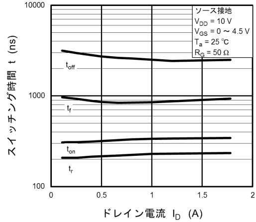
図 8.8 t - I_D
