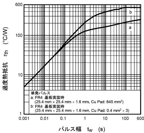
図 7.11 r_{th} - t_w
