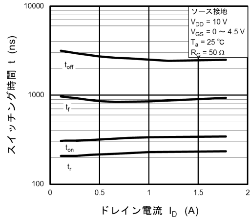
図 7.8 t - I_D
