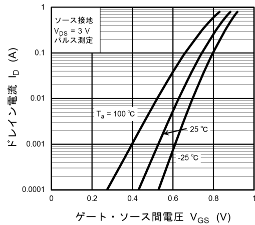
図 7.2 I_D - V_{GS}
