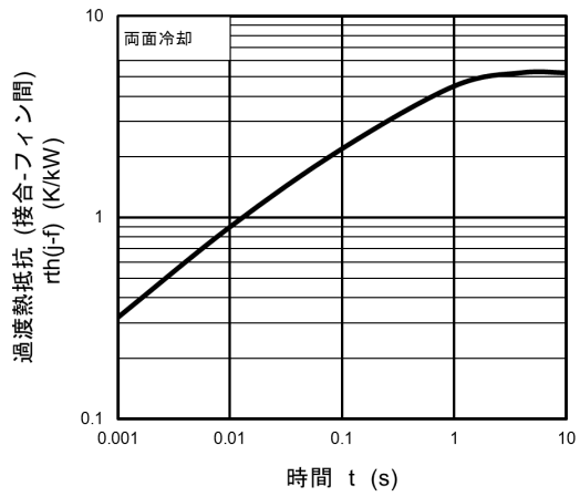
図 7.10 r_{th(j-f)} - t(\text{保証値})
