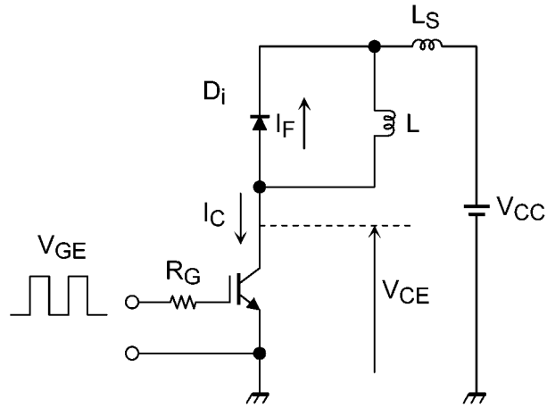
図 6.1 測定回路
