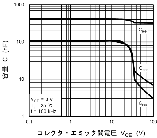
図 7.3 C_{ies}, C_{oes}, C_{res} - V_{CE}
