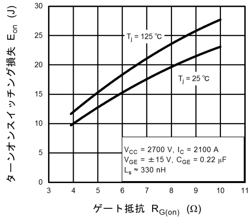
図 7.8 E_{on} - R_{G(on)}
