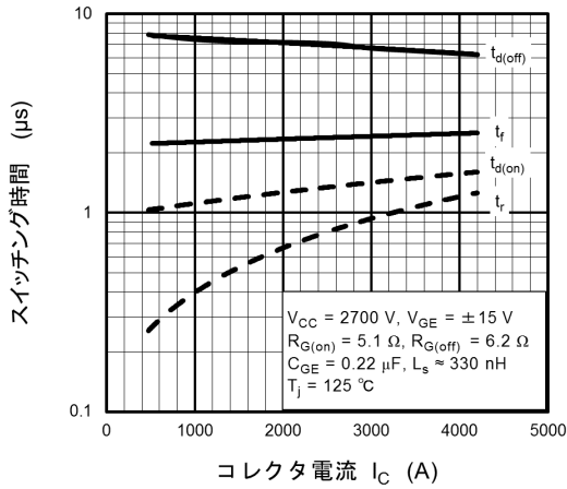
図 7.7 t_{d(off)}, t_r, t_{d(on)}, t_r - I_C
