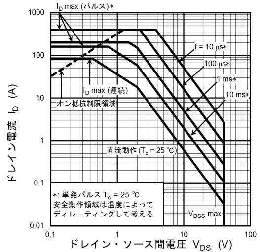
図 8.15 安全動作領域 (最大値 (保証値))
