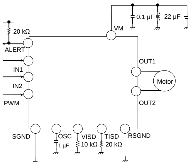
(a) ISD、TSD 自動復歸型回路例
