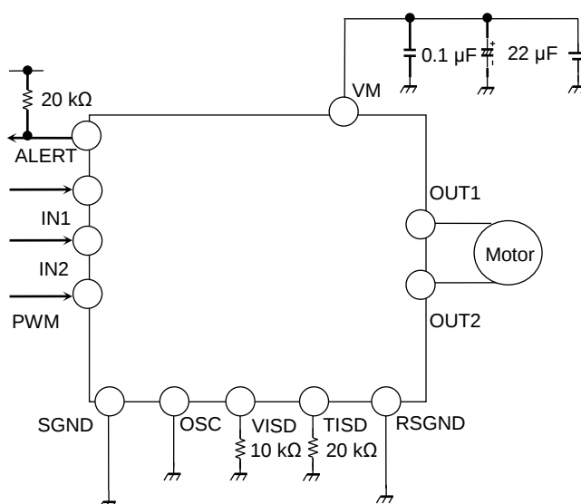
(b) ISD、TSD 他動復歸型回路例
