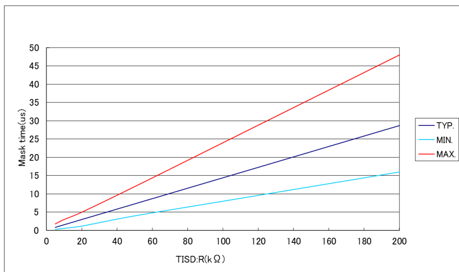
TISD 端子の外付け抵抗値 – ISD マスク時間の関係(参考値)
