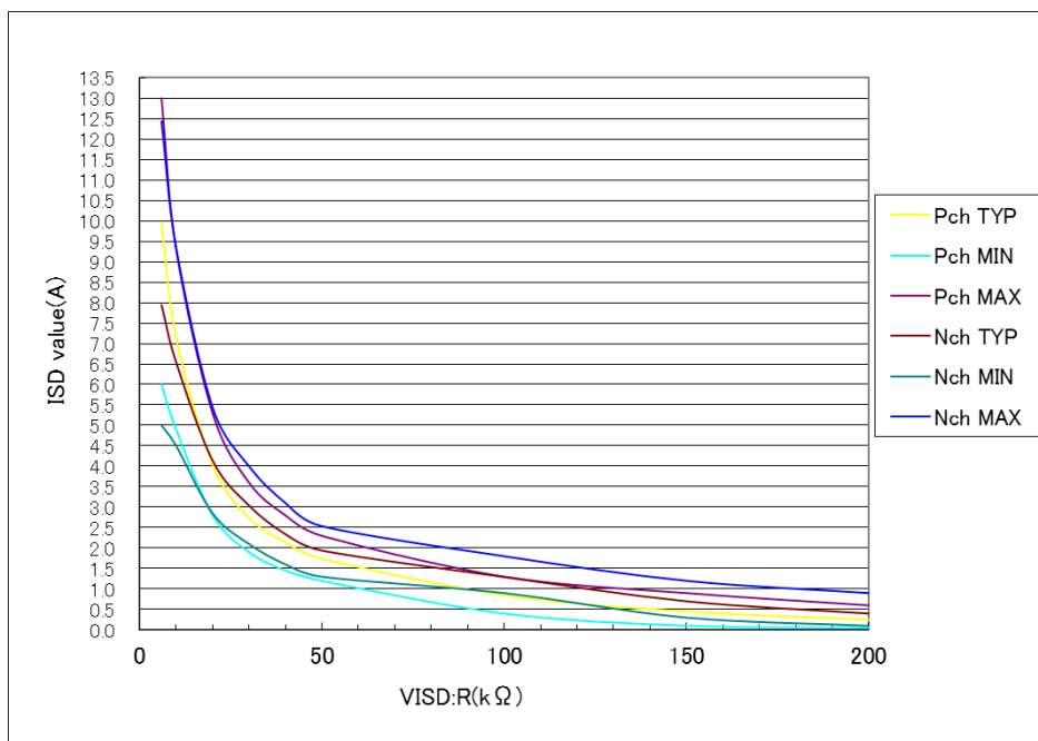
VISD 端子の外付け抵抗値 – ISD 検出電流値の関係(参考値)
