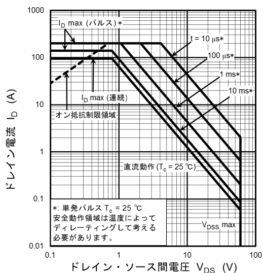
図 8.16 安全動作領域 (最大値 (保証値))
