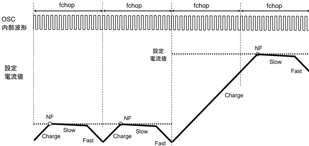
図 6.15 Charge 期間が fchop 1 周期以上の場合
