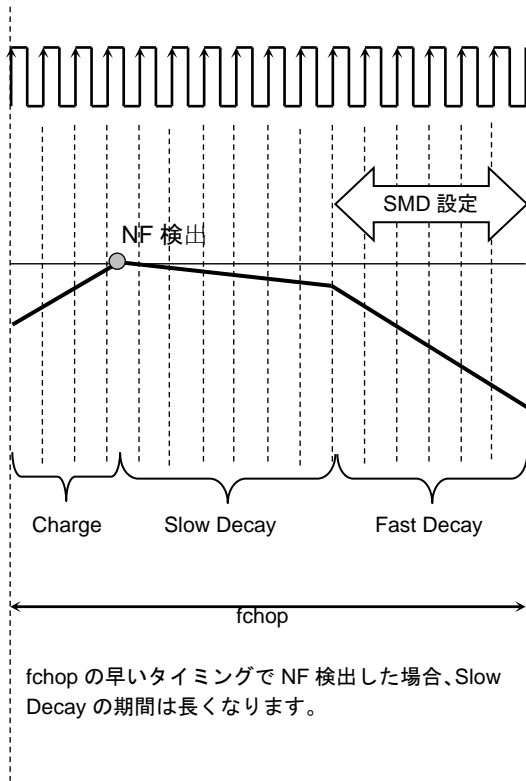
図 6.11 定電流 PWM 動作の各時間 (1)
