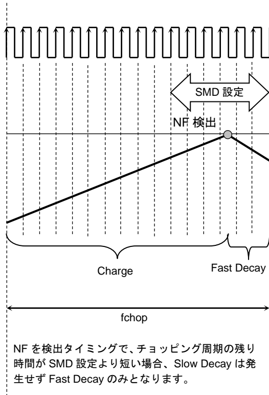
図 6.13 定電流 PWM 動作の各時間 (3)
