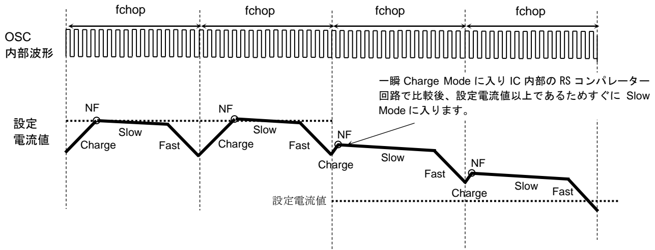
図 6.16 設定電流値が減少方向の場合
