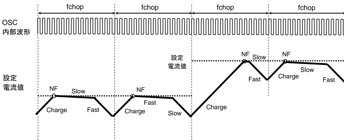
図 6.14 設定電流値が増加方向の場合
