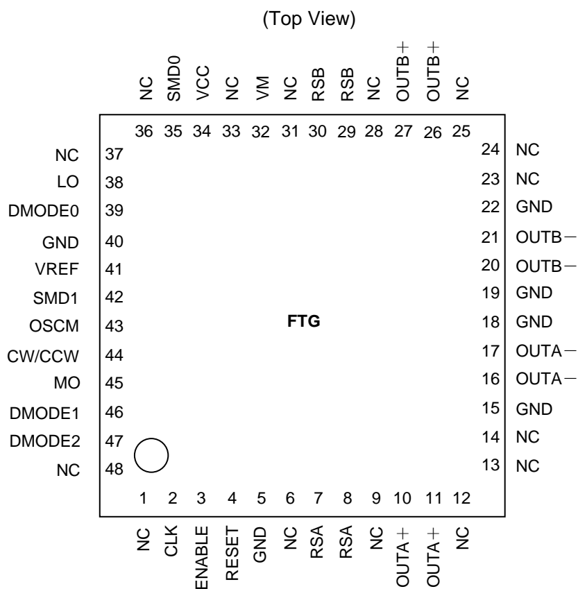
図 4.1 端子配置図
