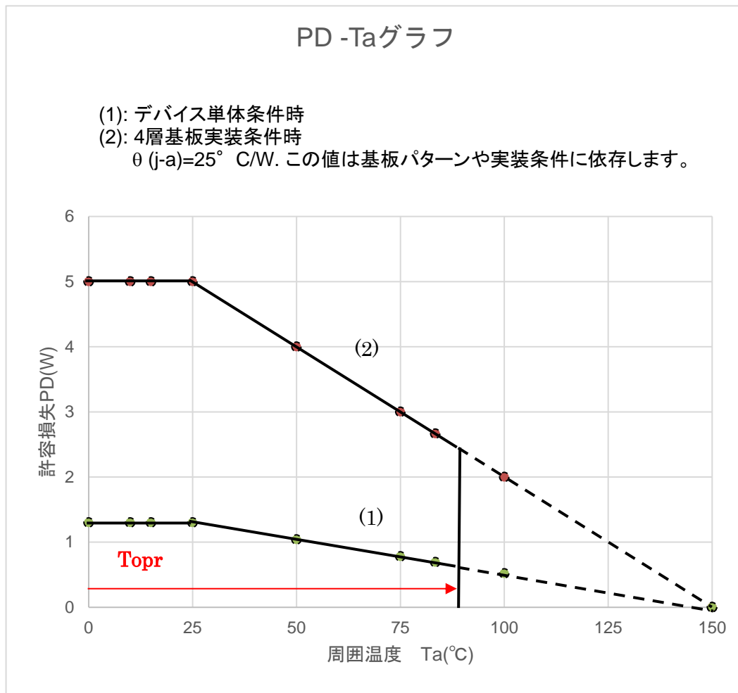
図7 PD - Ta (パッケージの許容損失)
