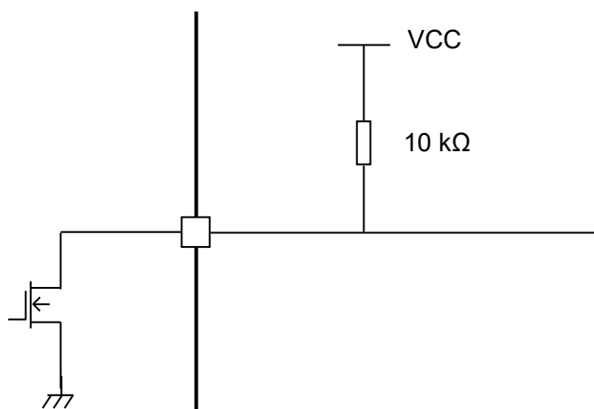
図 6.8 LO 端子
