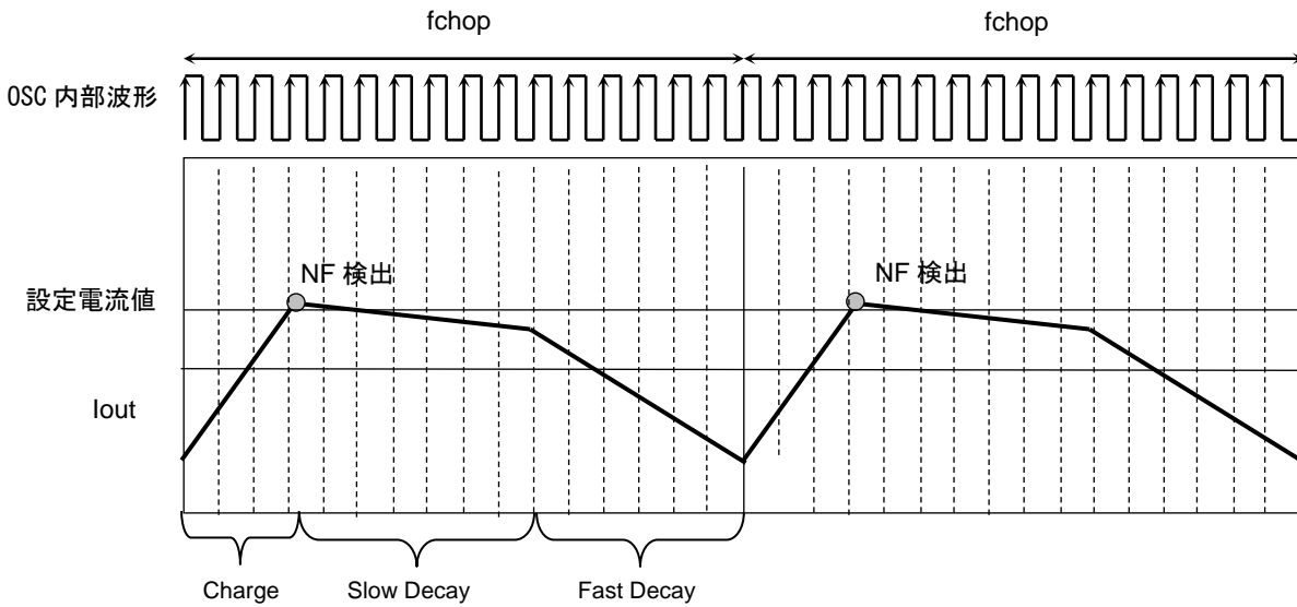
図 6.10 Mixed Decay の波形
