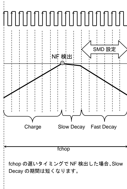
図 6.12 定電流 PWM 動作の各時間 (2)
