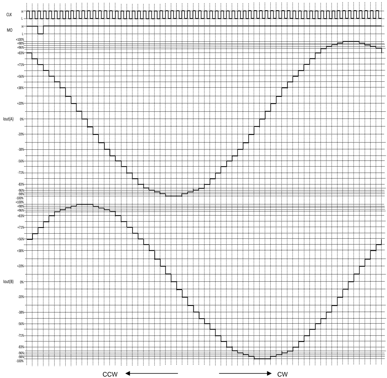
図 6.6 4W1-2 相励磁設定
