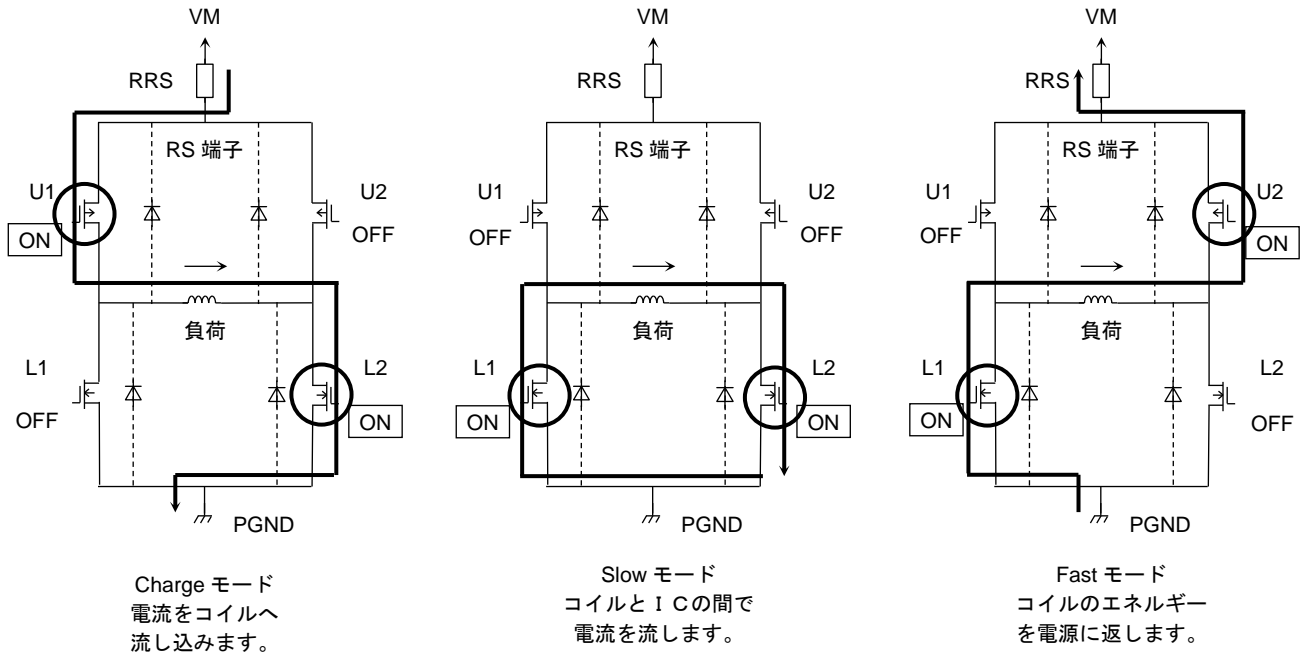
図 6.17 出力段トランジスタ動作モード
