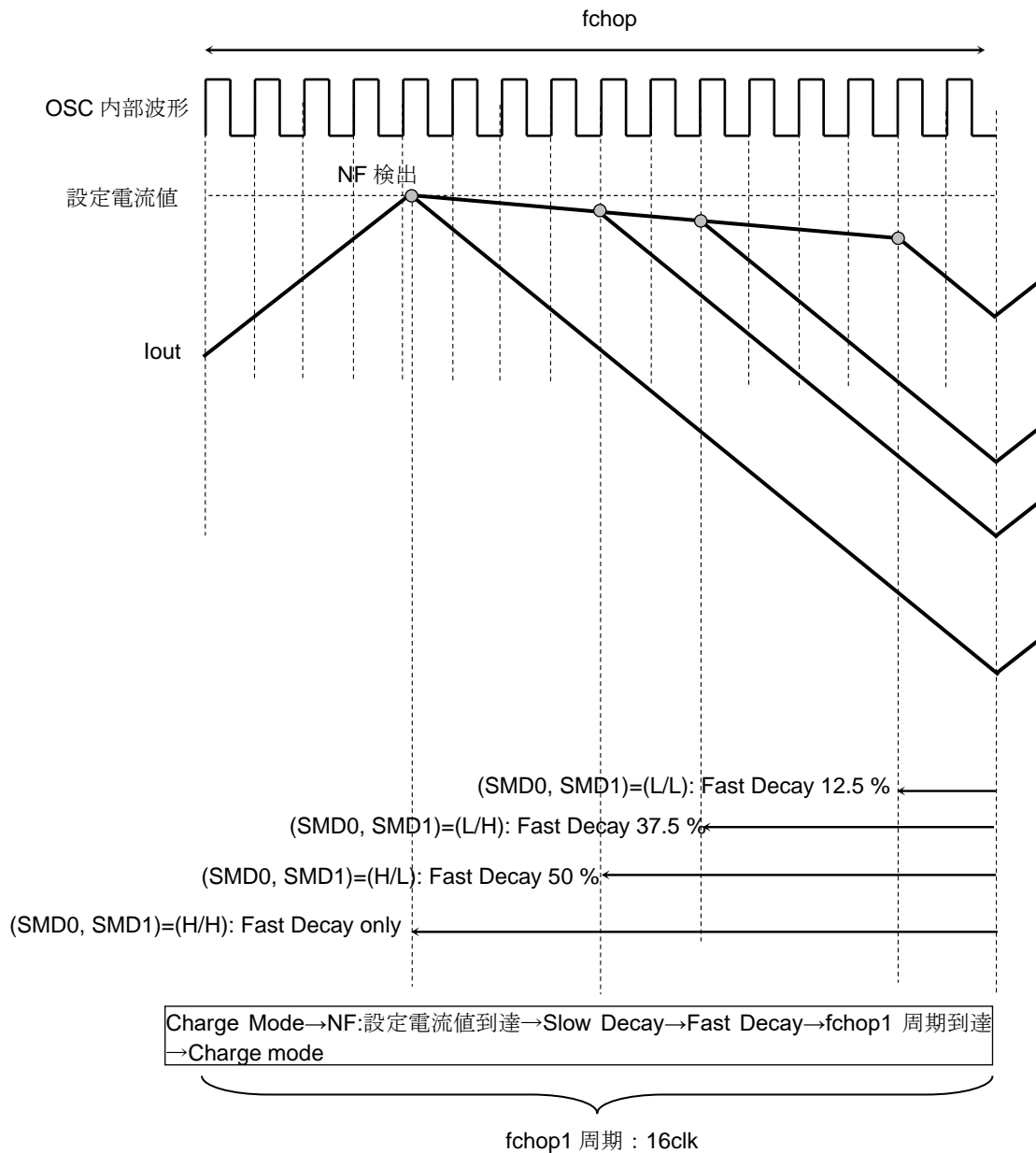
図 6.9 Selectable Mixed Decay
