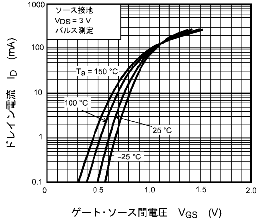
図 7.2 I_D - V_{GS}
