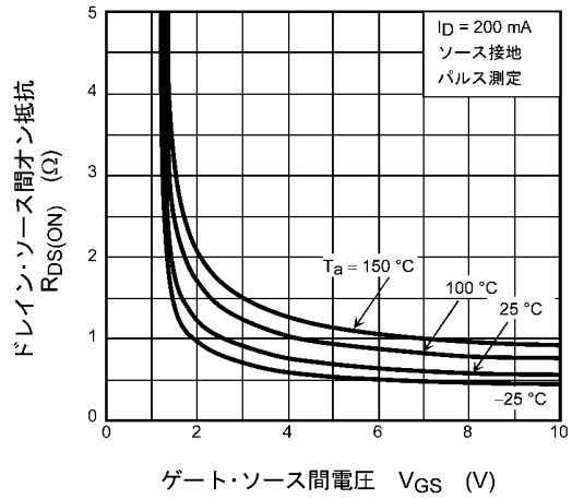
図 7.4 R_{DS(ON)} - V_{GS}
