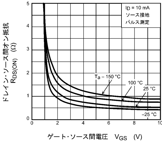
図 7.3 R_{DS(ON)} - V_{GS}
