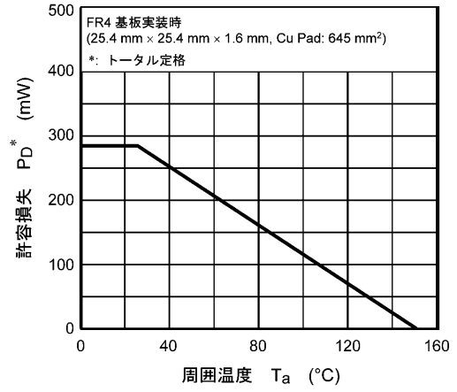
図 7.14 P_D - T_a
