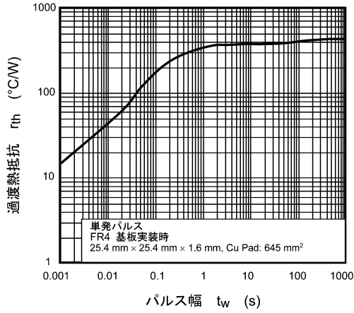
図 7.13 r_{th} - t_w
