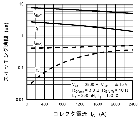
図 7.12 t_{d(off)}, t_f, t_{d(on)}, t_r - I_C
