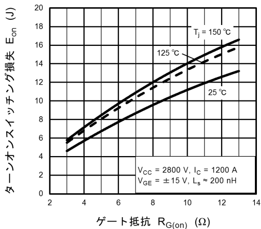
図 7.9 E_{on} - R_{G(on)}
