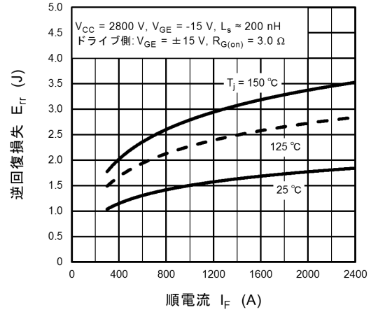
図 7.8 E_{rr} - I_F
