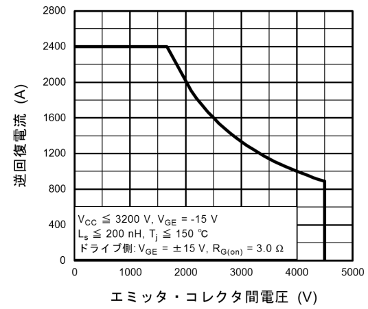
図 7.16 RRSOA (保証値)
