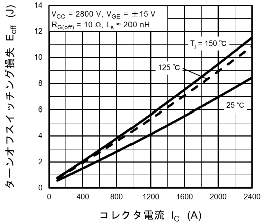
図 7.7 E_{off} - I_C
