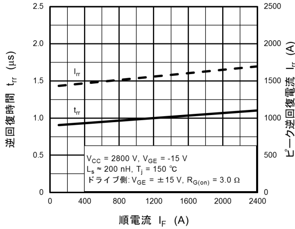
図 7.13 t_r, I_r - I_F
