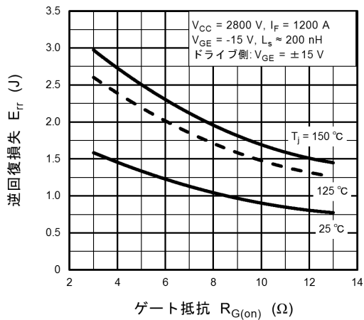
図 7.11 E_{rr} - R_{G(on)}
