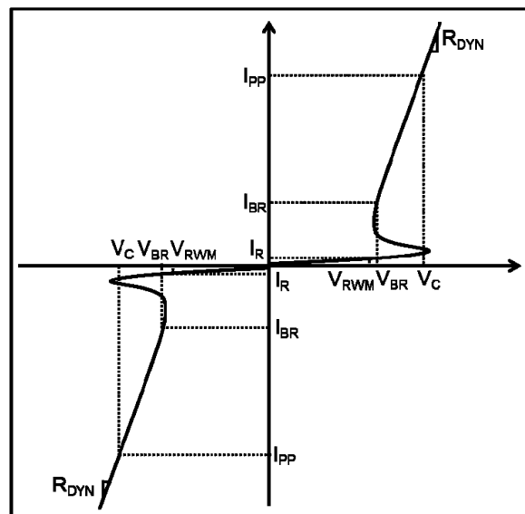
図 7.1 電気的特性の定義
