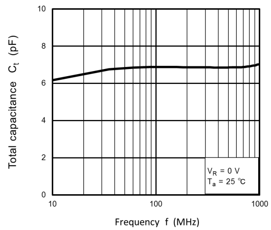
図 8.4 C_t - f
