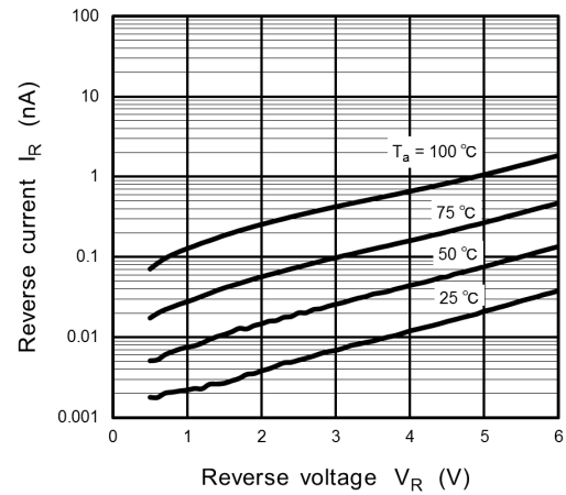
図 8.2 I_R - V_R
