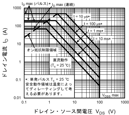
図 8.16 安全動作領域 (最大値 (保証値))
