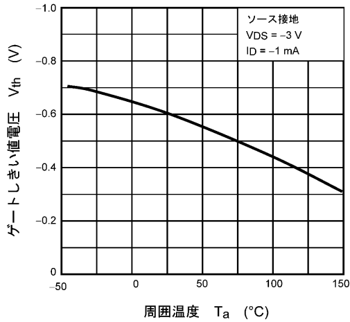
図 7.7 V_{th} - T_a
