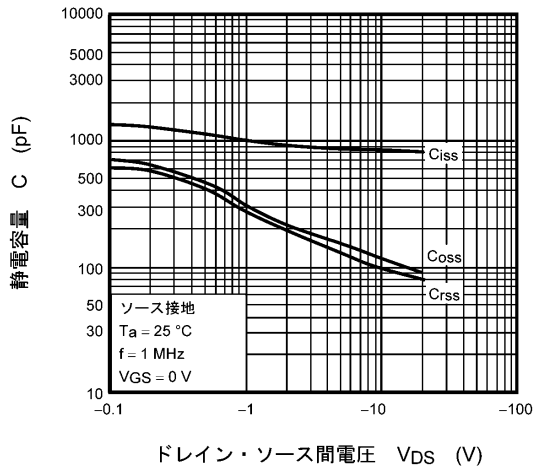
図 7.9 C - V_{DS}
