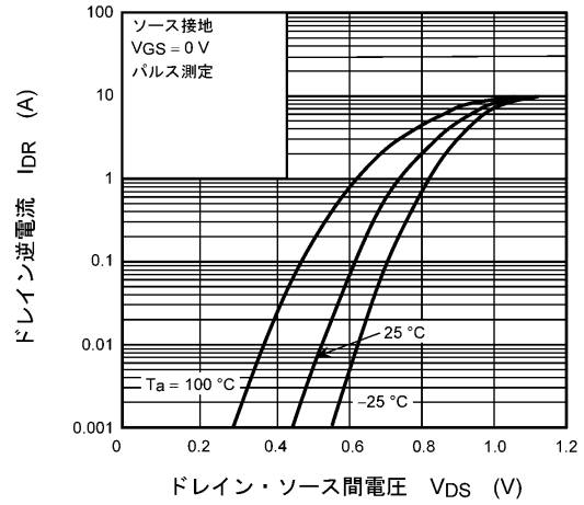
図 7.8 I_{DR} - V_{DS}
