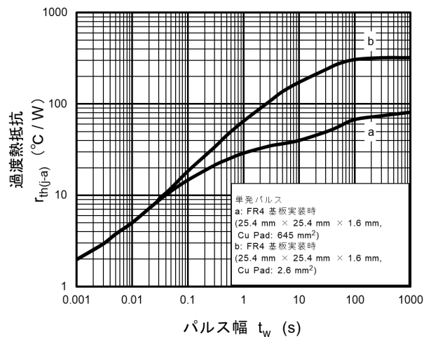
図 8.12 r_{th(j-a)} - t_w
