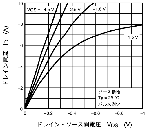
図 7.1 I_D - V_{DS}
