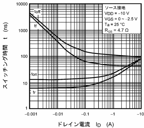
図 7.11 t - I_D
