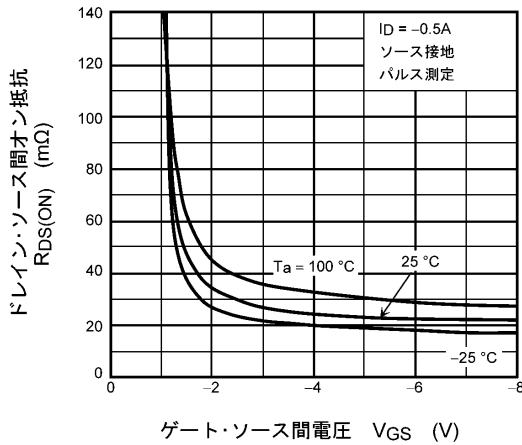
図 8.3 R_{DS(ON)} - V_{GS}
