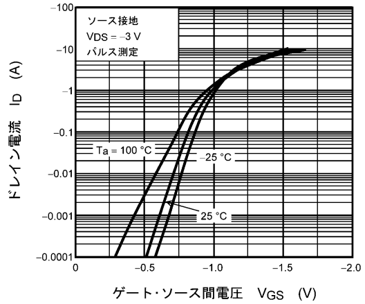
図 8.2 I_D - V_{GS}
