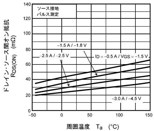
図 7.6 R_{DS(ON)} - T_a
