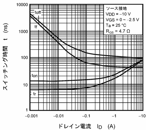
図 8.11 t - I_D
