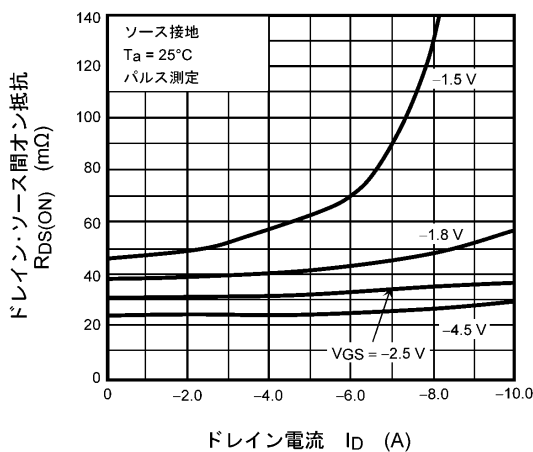
図 7.5 R_{DS(ON)} - I_D
