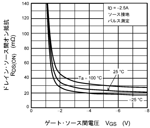
図 7.4 R_{DS(ON)} - V_{GS}
