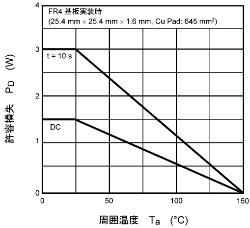
図 8.13 P_D - T_a
