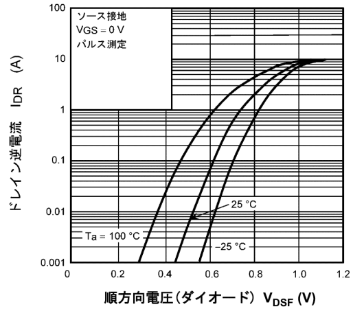
図 8.8 I_{DR} - V_{DSF}
