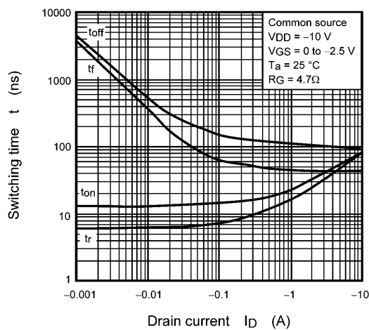
Fig. 7.11 t - I_D
