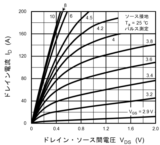
図 8.2 I_D - V_{DS}
