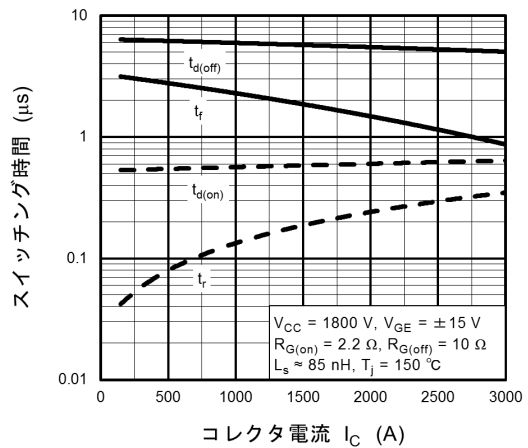
図 7.12 スイッチング時間 - I_C
