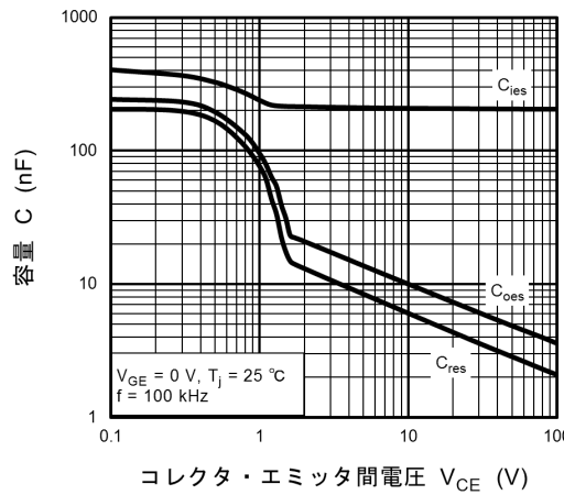
図 7.4 容量 - V_{CE}
