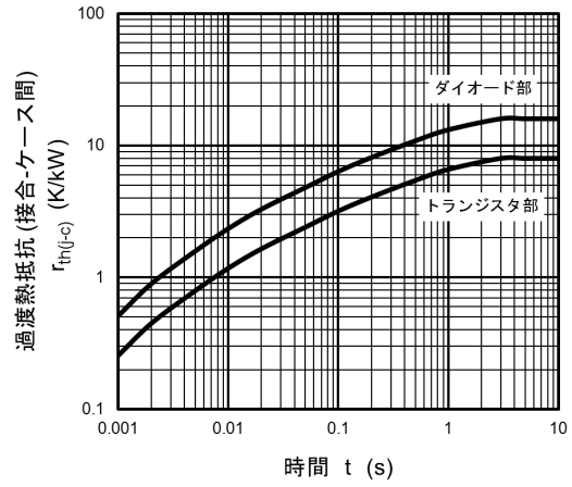
図 7.14 r_{th(j-c)} - t (保証値)
