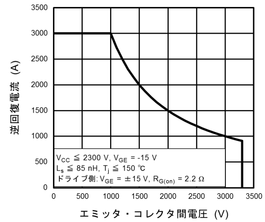
図 7.16 RRSOA(保証値)
