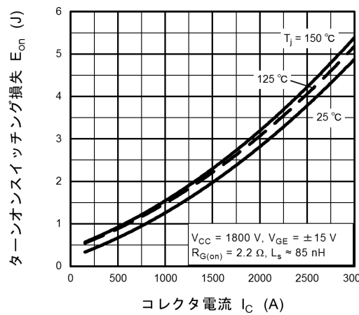
図 7.6 E_{on} - I_c
