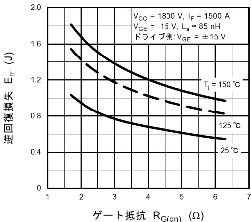
図 7.11 E_{rr} - R_{G(on)}
