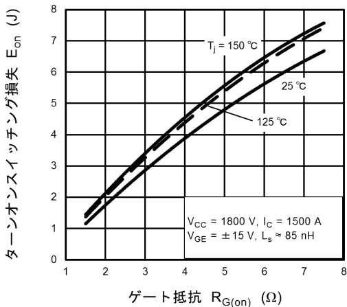
図 7.9 E_{on} - R_{G(on)}
