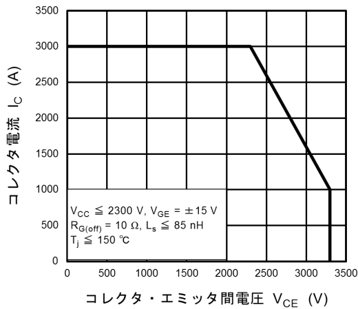
図 7.15 RBSOA(保証値)
