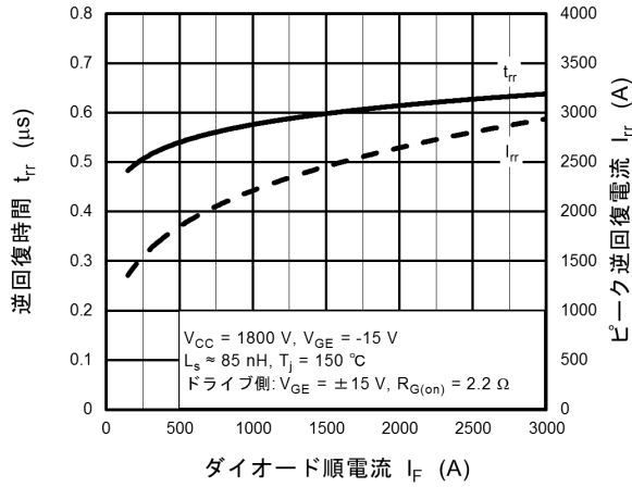
図 7.13 t_{rr}, I_{rr} - I_F
