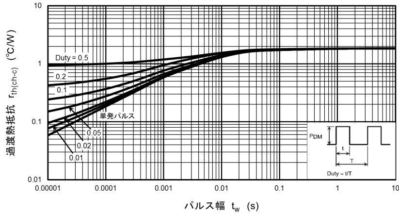
図 8.13 r_{th(ch-c)} - t_w (最大値 (保証値))
