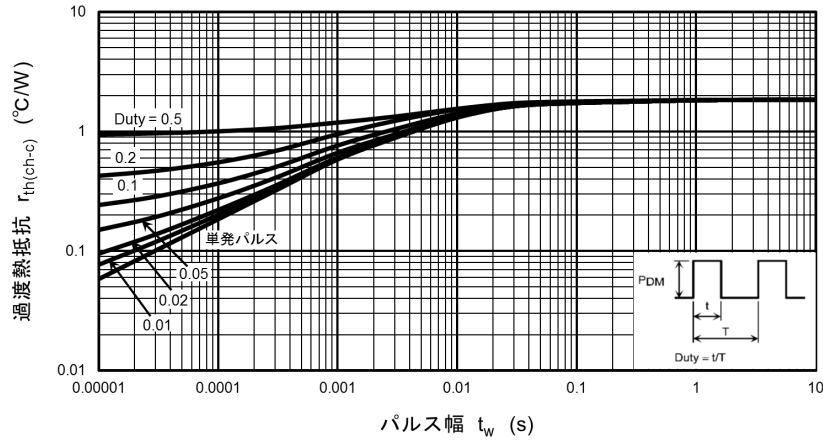
図 8.13 r_{th(ch-c)} - t_w (最大値 (保証値))
