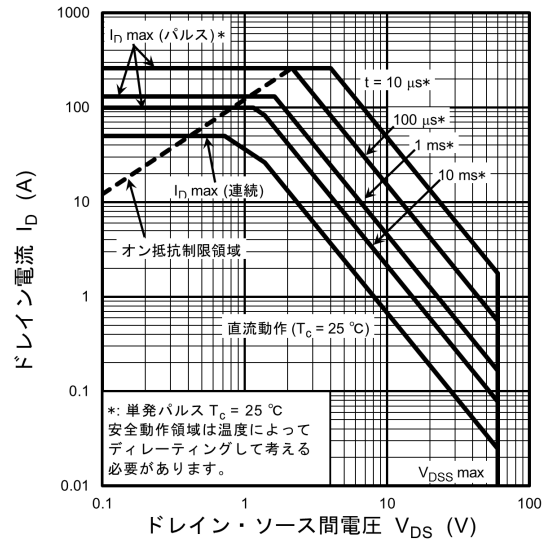
図 8.15 安全動作領域 (最大値 (保証値))
