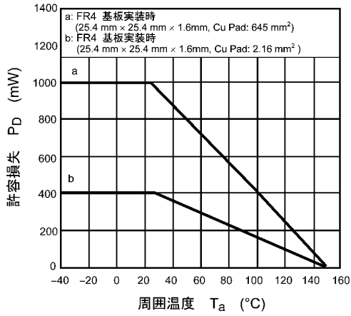
図 7.13 P_D - T_a
