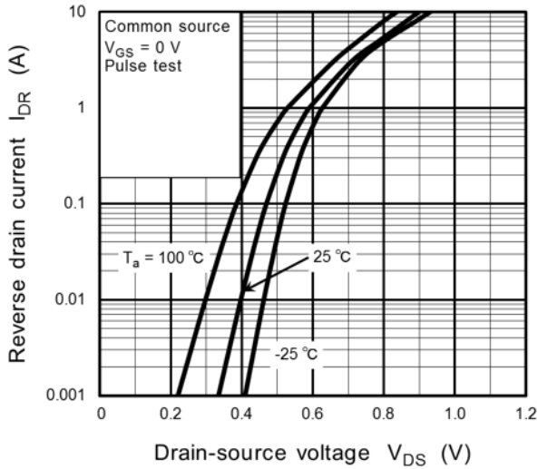
Fig. 7.7 I_{DR} - V_{DS}
