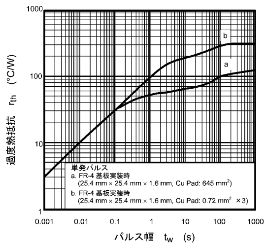
図 8.13 r_{th} - t_w
