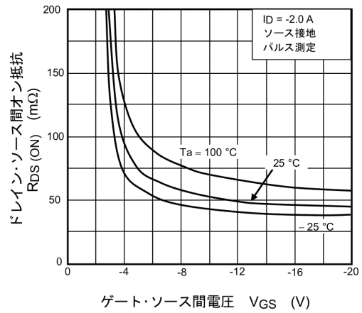
図 8.4 R_{DS(ON)} - V_{GS}
