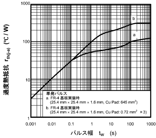
図 8.13 r_{th(j-a)} - t_w
