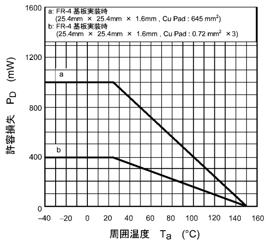
図 8.14 P_D - T_a
