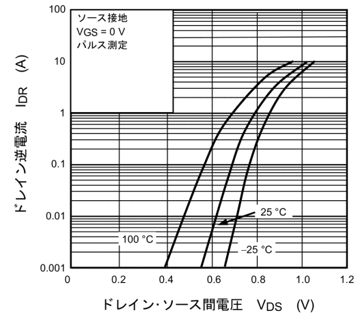
図 8.12 I_{DR} - V_{DS}
