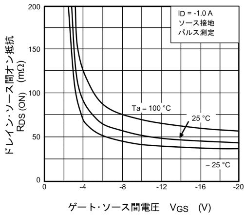
図 8.3 R_{DS(ON)} - V_{GS}
