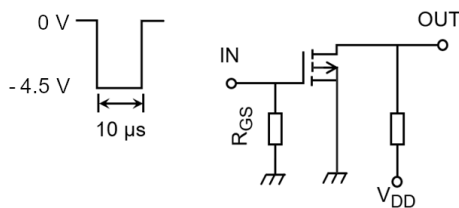
図 6.3.1 スwitching時間の測定回路
