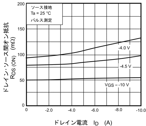
図 8.5 R_{DS(ON)} - I_D
