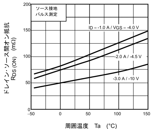
図 8.6 R_{DS(ON)} - T_a
