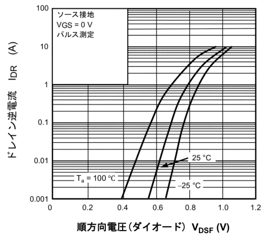
図 8.12 I_{DR} - V_{DSF}
