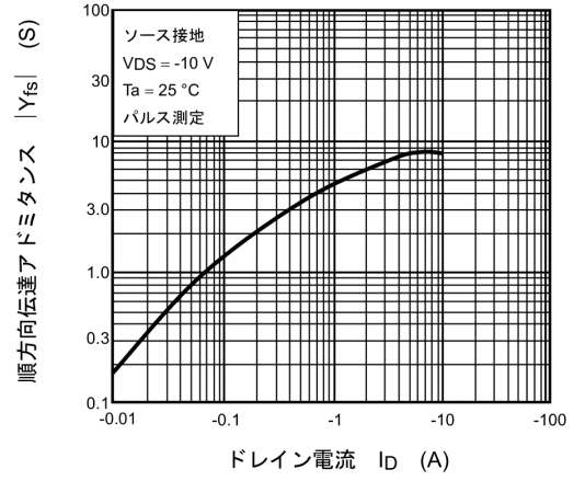
図 8.8 |Y_{fs}| - I_D
