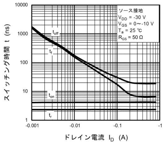
図 8.10 t - I_D
