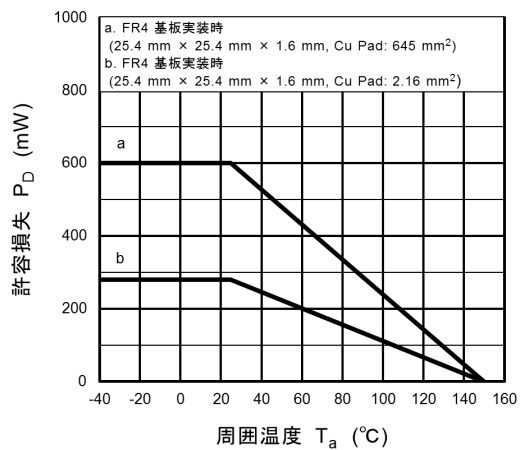
図 7.13 P_D - T_a
