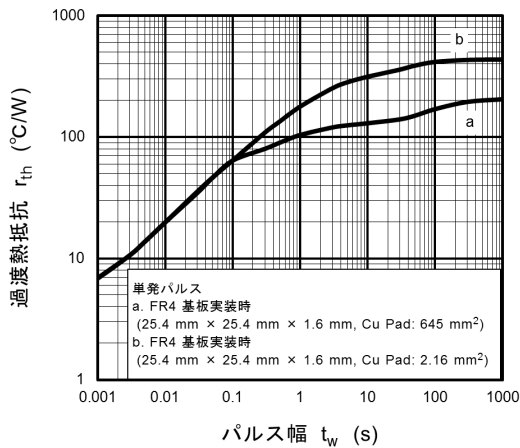
図 7.11 r_{th} - t_w
