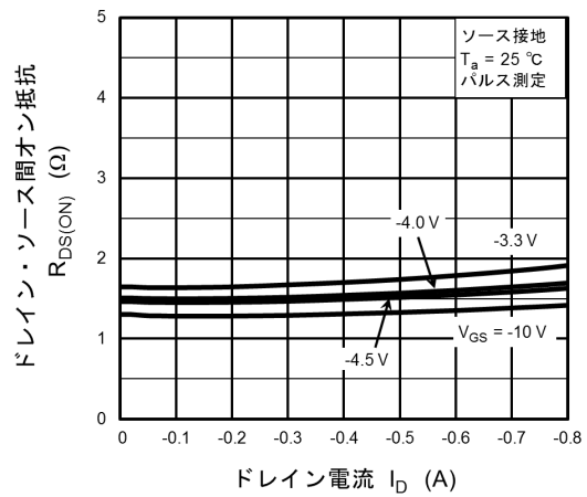
図 7.4 R_{DS(ON)} - I_D
