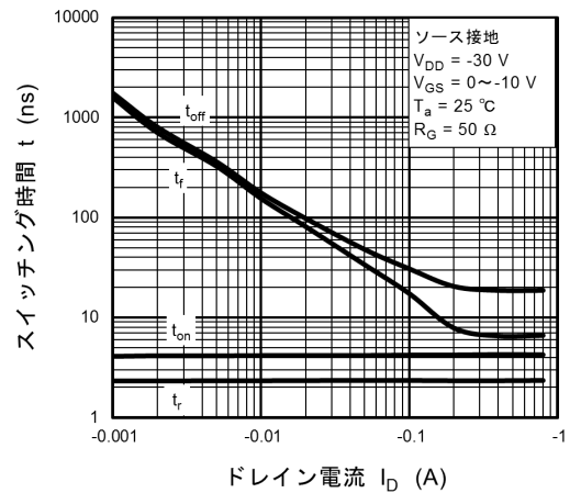
図 7.10 t - I_D
