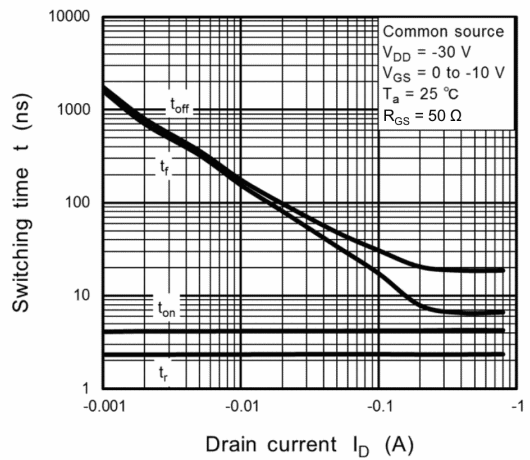
Fig. 8.10 t - I_D
