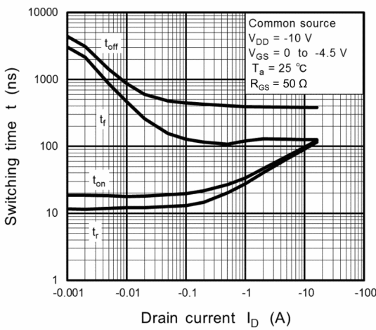
Fig. 8.9 t - I_D
