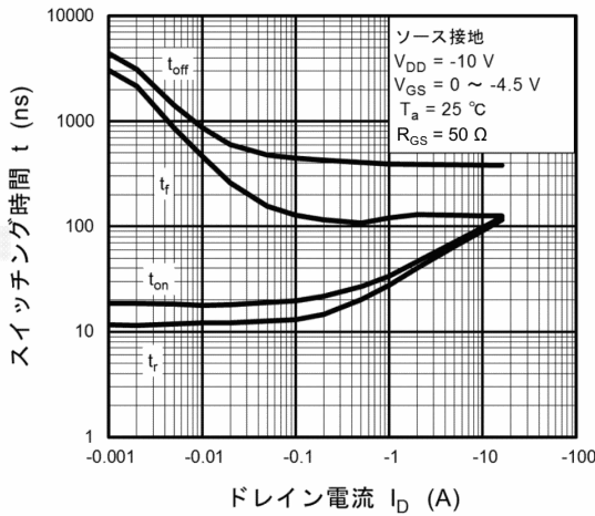
図 8.9 t - I_D
