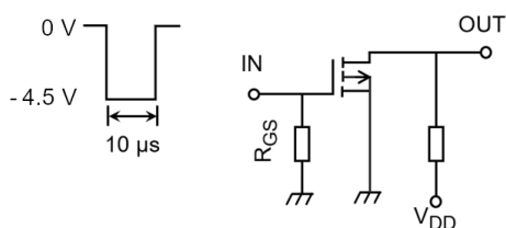
図 6.3.1 スイッチング時間の測定回路
