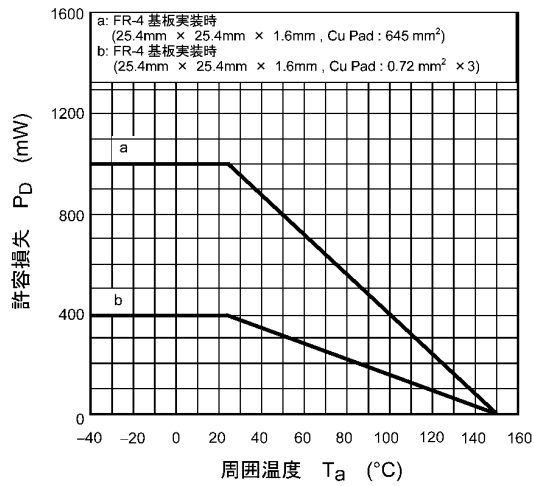
図 8.13 P_D - T_a
