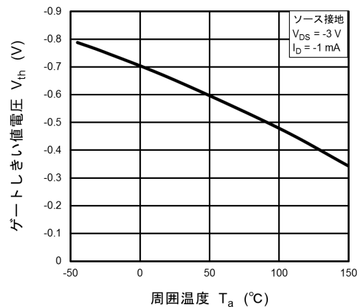
図 7.6 V_{th} - T_a
