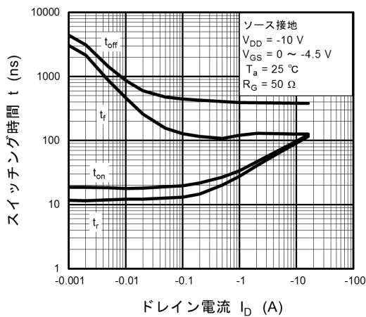
図 7.9 t - I_D
