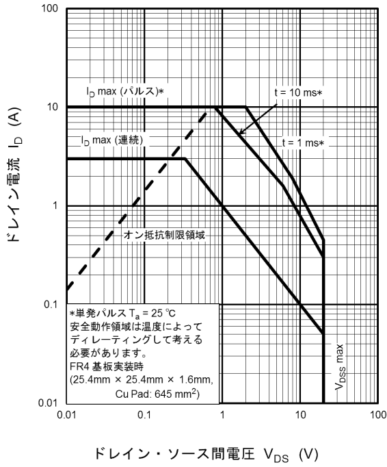
図 8.13 安全動作領域
