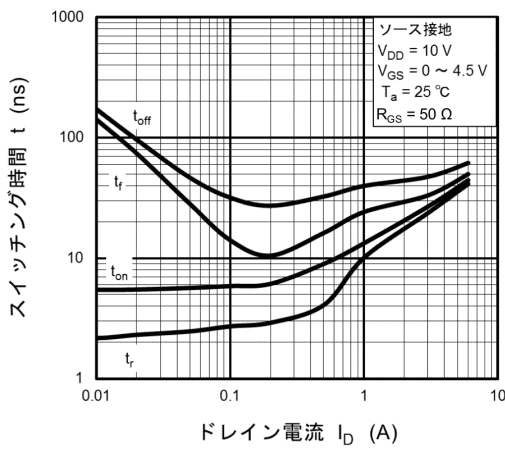
図 8.9 t - I_D
