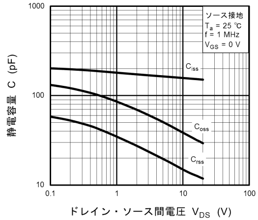
図 8.8 C - V_{DS}
