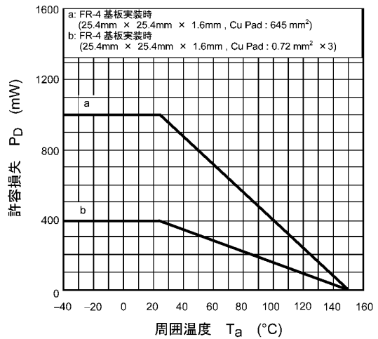
図 8.12 P_D - T_a
