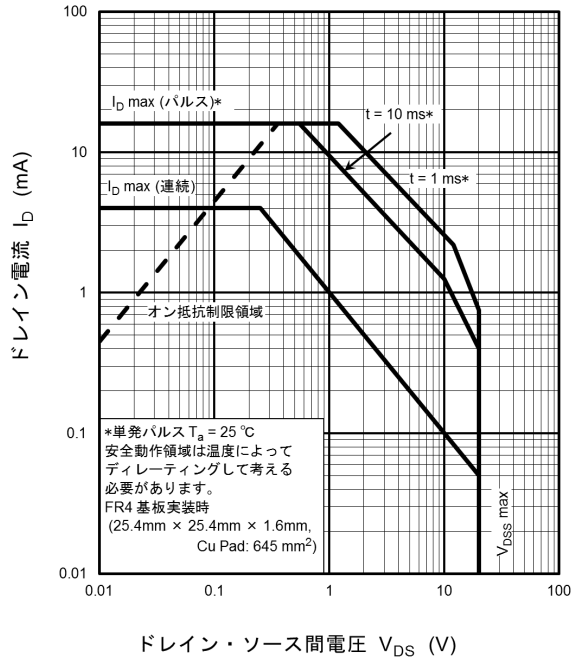
図 7.13 安全動作領域
