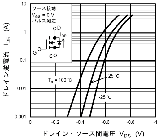
図 7.7 I_{DR} - V_{DS}
