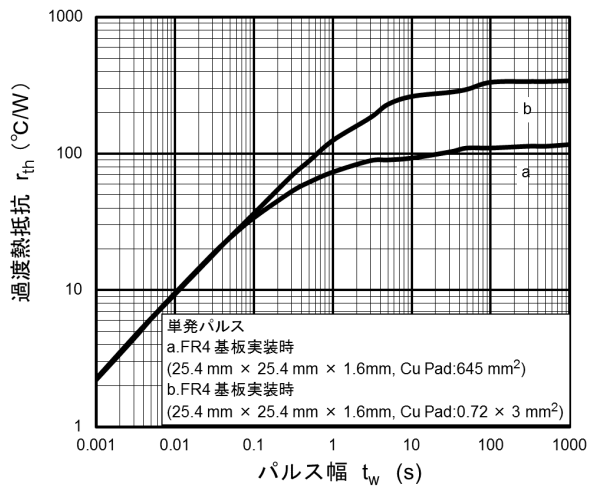
図 7.11 r_{th} - t_w
