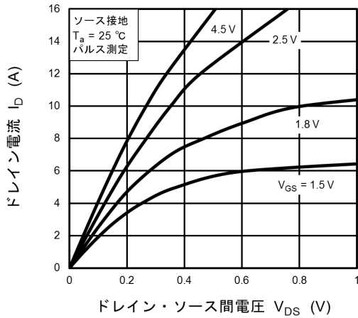
図 7.1 I_D - V_{DS}
