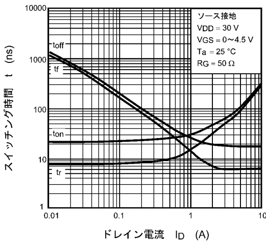
図 7.9 t - I_D
