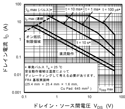
図 7.11 安全動作領域
