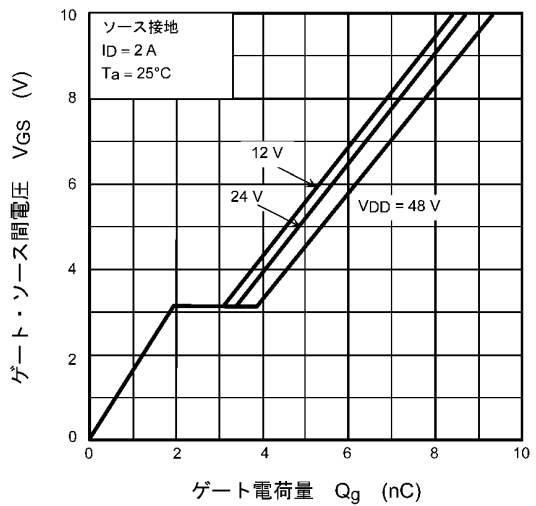
図 7.10 ダイナミック入力特性
