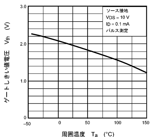
図 7.6 V_{th} - T_a
