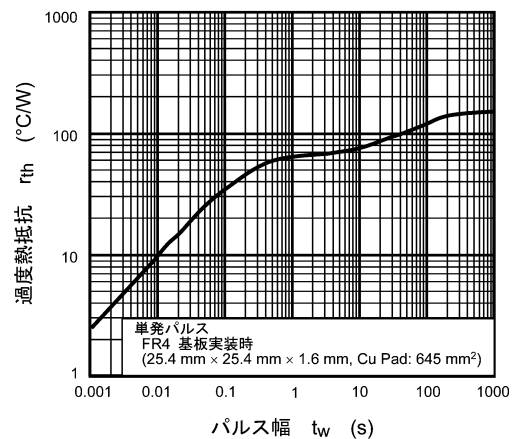
図 7.12 r_{th} - t_w
