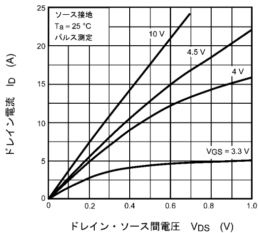
図 7.1 I_D - V_{DS}
