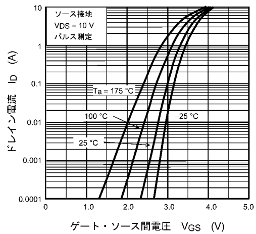
図 8.2 I_D - V_{GS}
