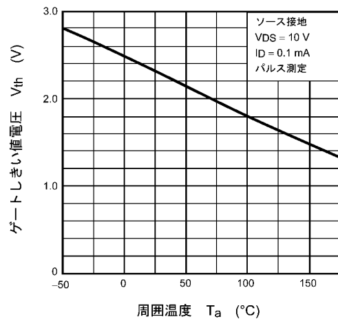
図 7.6 V_{th} - T_a
