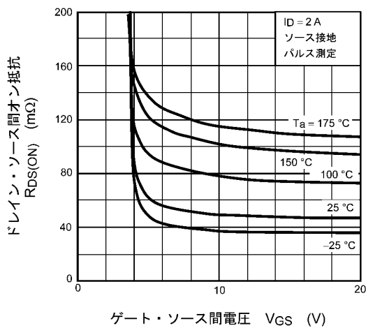
図 8.3 R_{DS(ON)} - V_{GS}
