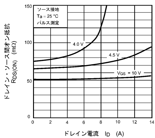
図 8.4 R_{DS(ON)} - I_D
