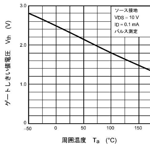
図 8.6 V_{th} - T_a
