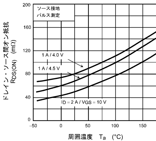
図 7.5 R_{DS(ON)} - T_a
