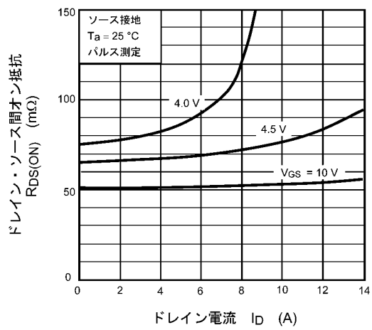
図 7.4 R_{DS(ON)} - I_D
