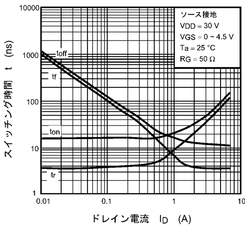
図 7.9 t - I_D
