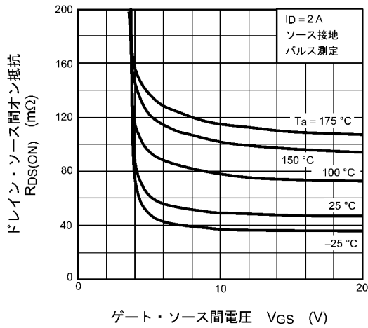
図 7.3 R_{DS(ON)} - V_{GS}
