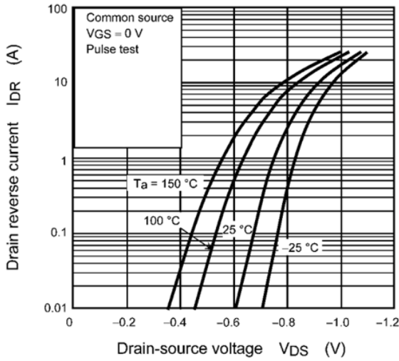
Fig. 8.7 I_{DR} - V_{DS}
