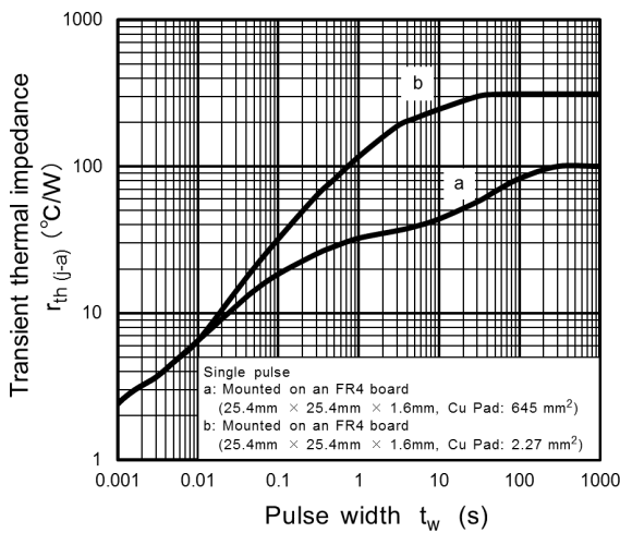
Fig. 8.11 r_{th} - t_w
