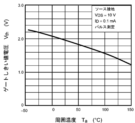
図 9.6 V_{th} - T_a
