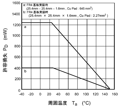
図 9.13 P_D - T_a
