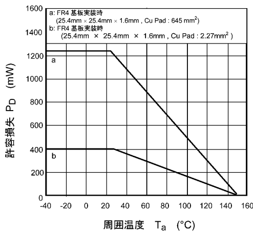
図 8.11 P_D - T_a
