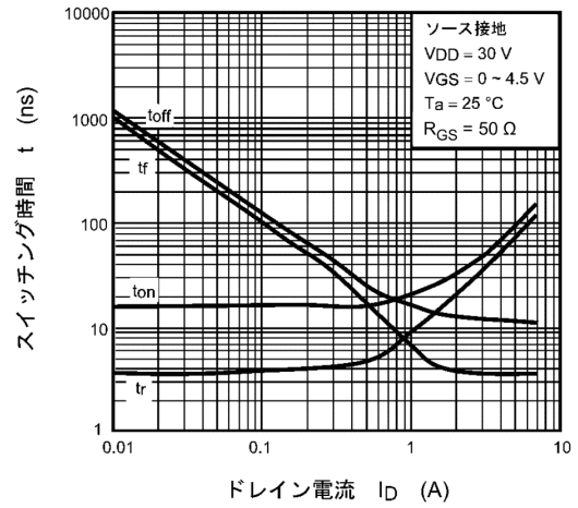
図 9.4 t - I_D
