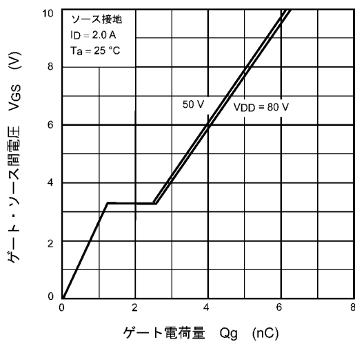
図 9.5 ダイナミック入力特性
