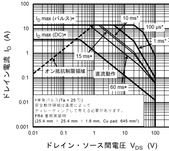
図 8.7 安全動作領域
