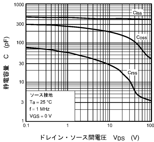
図 9.3 C - V_{DS}
