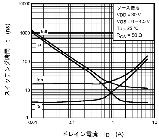
図 8.4 t - I_D
