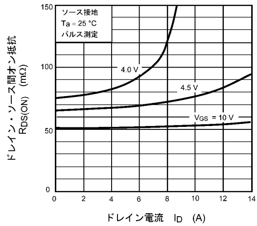
図 8.2 R_{DS(ON)} - I_D
