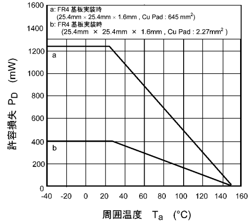
図 9.8 P_D - T_a
