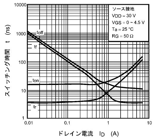
図 8.4 t - I_D
