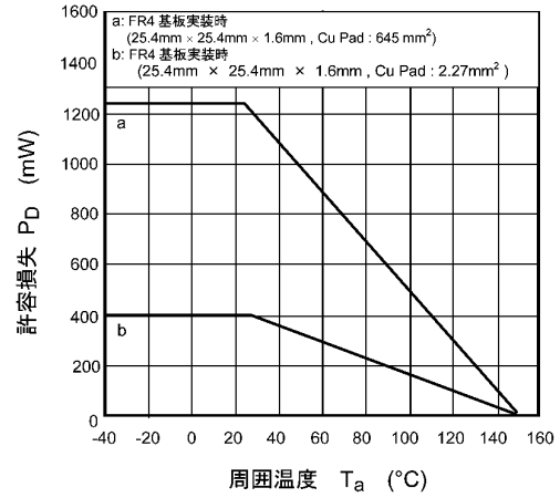
図 8.8 P_D - T_a
